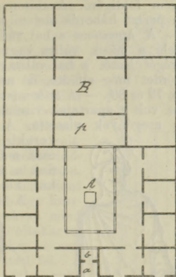
A görög ház alaprajza.
