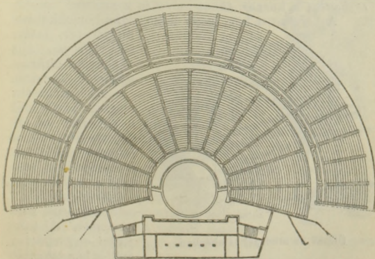
Az epidaurosí színház alaprajza.
