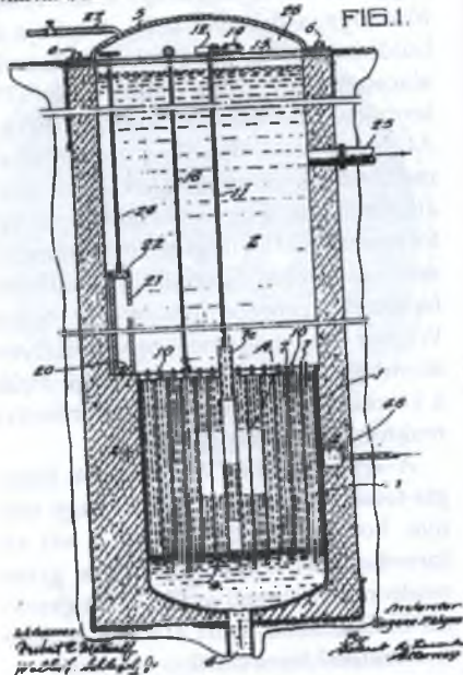
Wigner Jenő egyik tenyésztő-reaktor szabadalma
