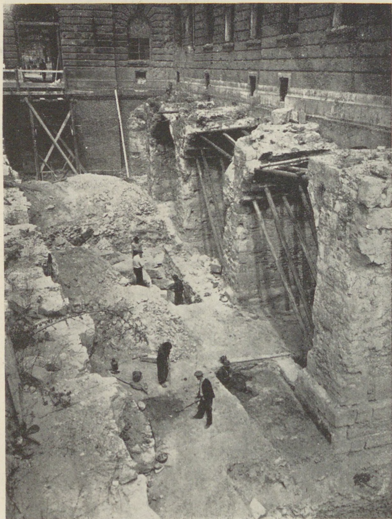
A Zsigmond palota Ny-i udvara az 1952-es feltárás közben
