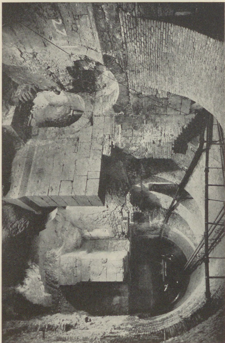
Az Anjou-palota Dunăra néző homlokzatának támpillérei a mai palota pincéjében
