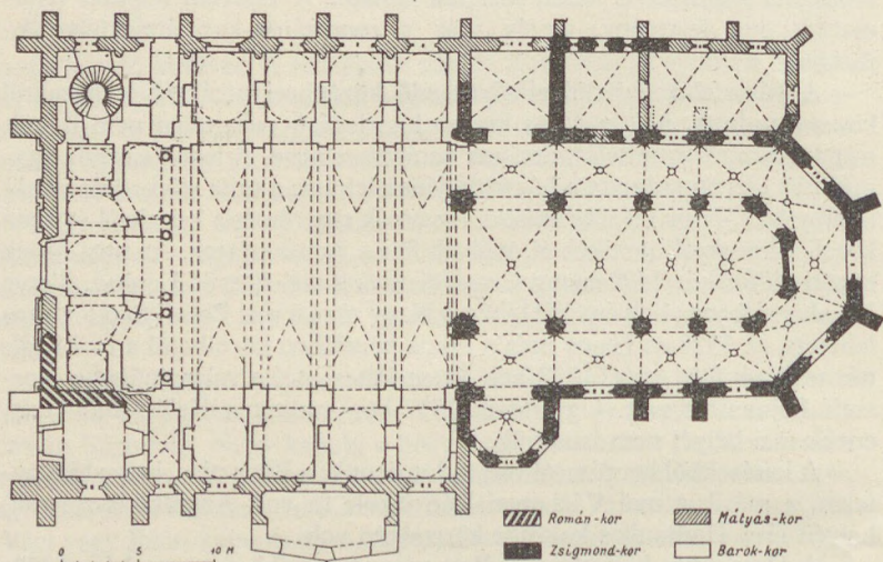
A Belvárosi templom alaprajza
