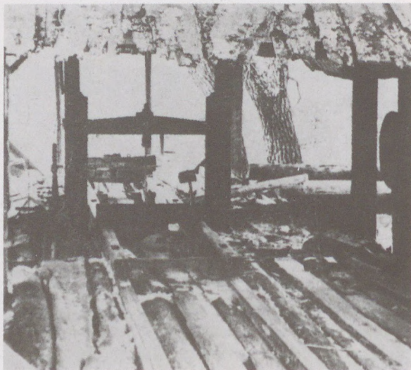
33. A fűrész szerkezete. MáL
