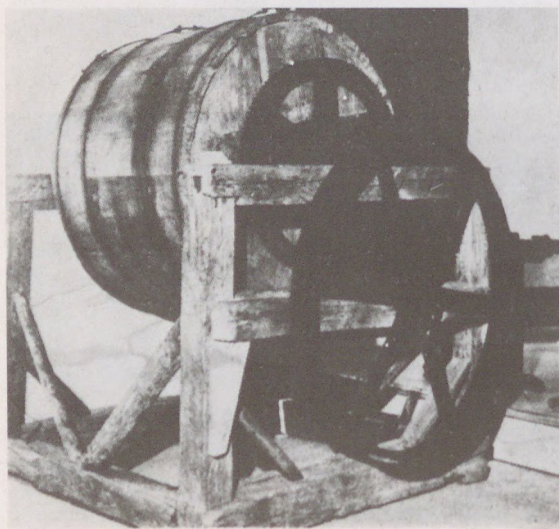
21. Tímár forgóhordó (a meszes bőrök öblítésére). BM
