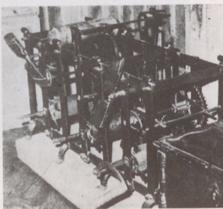
75. A gyergyószentmiklósi toronyóra szerkezete, 1861. BM
