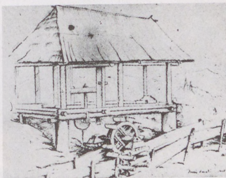
30. Egyszerű vízfűrész. Imets László rajza
