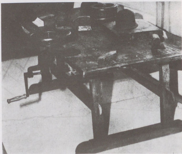
24. A kalaposság eszközei. BM
