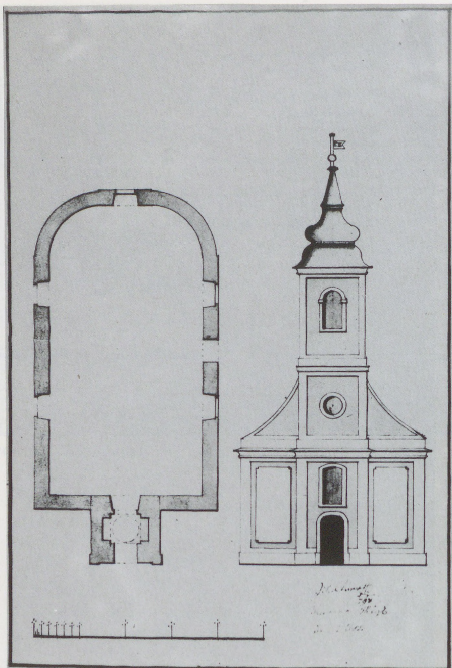
20. A sósvertikei templom homlokzat- és alaprajza, 1798
