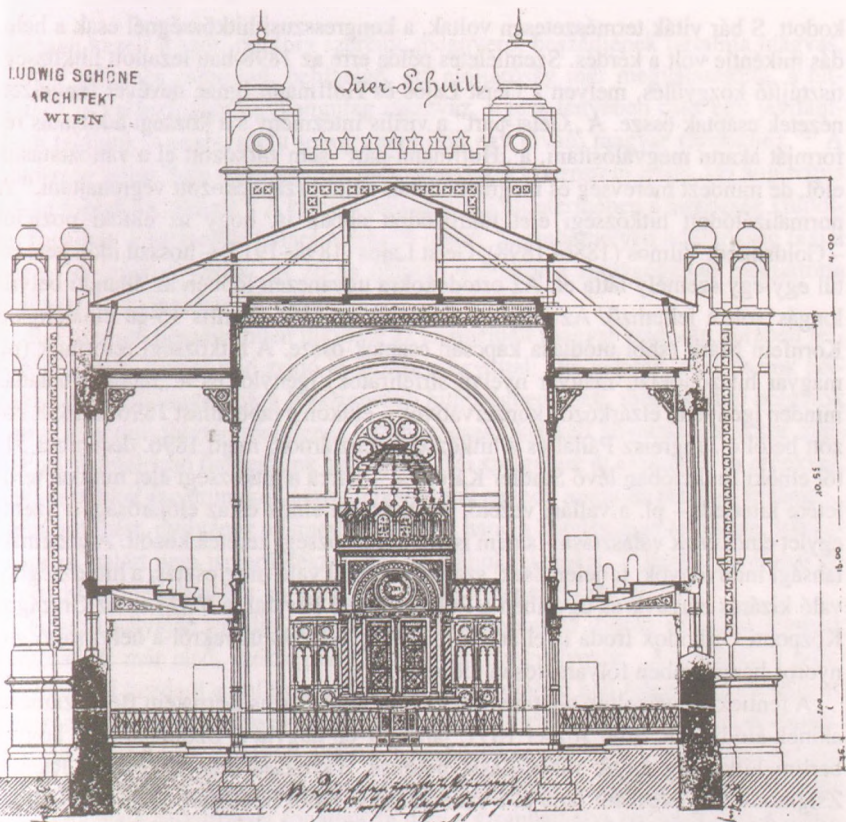
A szombathelyi kongresszusi izraelita hitközség zsinagógájának metszeti rajza a tóraszekrényvel
