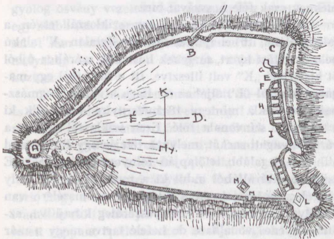
36. Brassóvár alaprajza.
