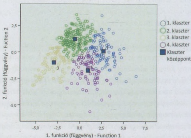
9. ábra: A klaszter centroidok ábrázolása a diszkriminanciafüggvények tükrében
