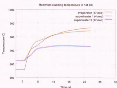
19. ábra. Maximális fűtőelem-burkolat hőmérsékletek a három forrócsatornában
