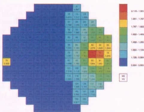
17. ábra. A kötegek relatív teljesítmény-növekedése a rúdkiöködés esetén
