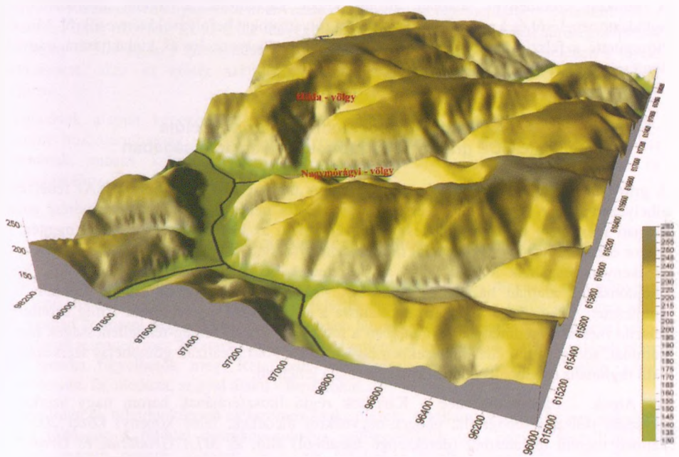
2. ábra. Digitális terepmodell a Nagymórággyi-völgy környezetének dombsági felszínéről
