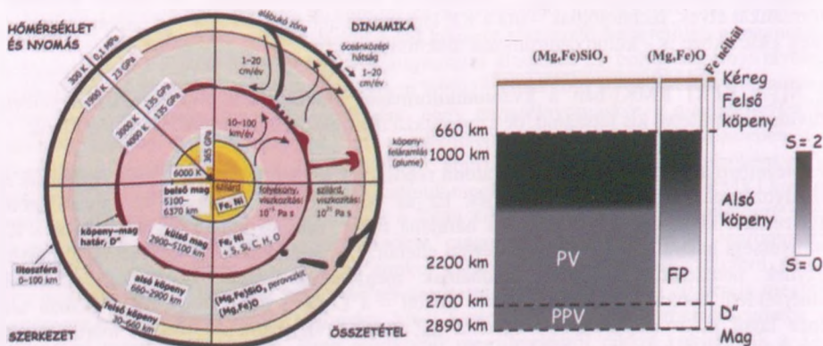
26. ábra. Balra: a Föld belseje főbb jellemzőinek összefoglalása. Jobbra: a \text{Fe}^{II} spinállapota az alsó köpeny ásványaiban. A téglalapok vastagsága az egyes ásványfajták mennyiségével arányos, a spinállapotot a színskála jelzi
