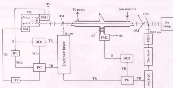
9. ábra. Impulzuslézerekkel működtetett reakciókinetikai berendezés a légkör kémiai folyamatainak laboratóriumi vizsgálatára
