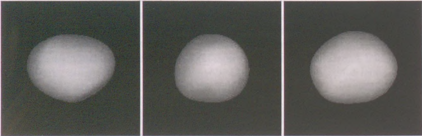
28. ábra. A 2867 Steins aszteroida háromdimenziós alakmodellje földi távcsövekkel megfigyelt 26 fénygörbe felhasználásával készült. A bal oldali és középső képen az egyenlítő síkjában látunk rá a kisbolygóra két, egymásra merőleges irányból. A jobb oldali képen az egyik pólusa felől nézzük a kis égitestet (kép: Rosetta OSIRIS kutatócsoport)
