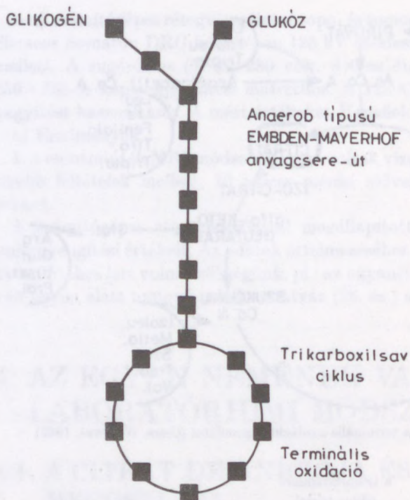
2. ábra. A glukóz energiát termelő lebontási folyamatának (oxidatív foszforilációjának) vázlata
