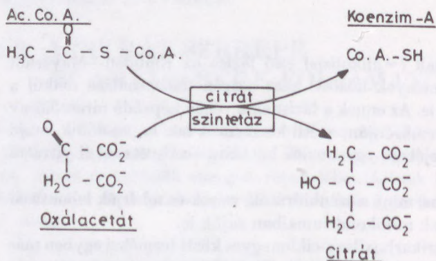
3. ábra. A citrát képződéséhez vezető kondenzációs folyamat (Orten, Neuhaus, 1982)
