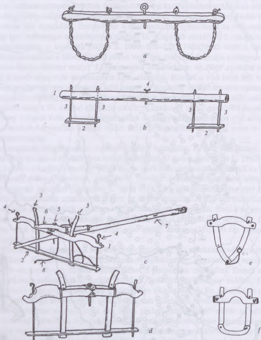
203. ábra. Járomfajták: a) íves marhajárom tölgy vesszőből csavart gúzzsal, Nyírgyulaj (Szabolcs vm.); b) küllős magyar iga. Részei: 1. felső igafa, 2. alsó igafa, 3. igaküllű, 4. igazszeg, Hetés (Zala vm.); c) ökrjárom tézslával. Részei: 1. járomfa, 2. alfa, 3. bélfá, 4. járompálca, 5. járomszeg, 6. rúdfő, 7. tézsula, 8. istráng, Mezőköbölkút (Kolozs vm.); d) bivalyjárom, Katona (Kolozs vm.); e) egyesjárom a mosoni németeknél (1950–60-as évek); f) egyesjárom (Nyugat-Dunántúl)
