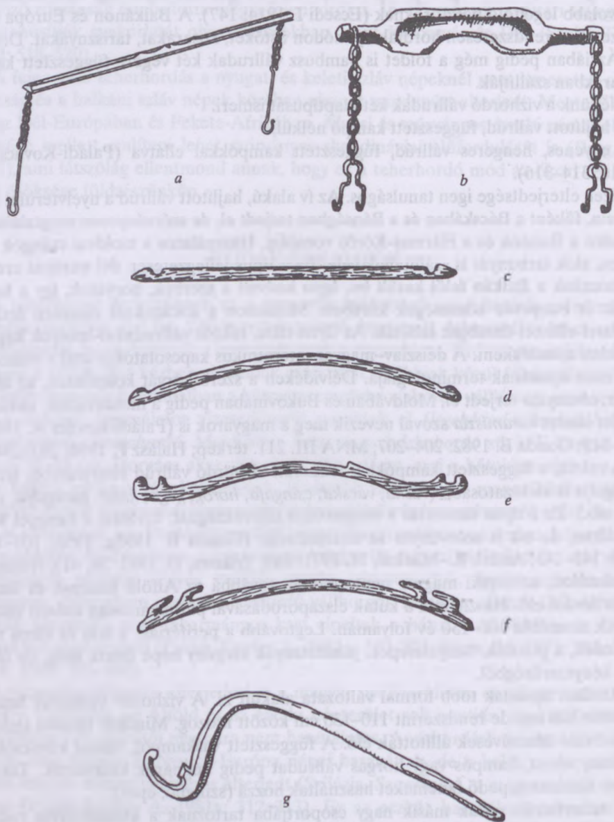
188. ábra. Teherhordó rudak: a) vízhordó rúd (1950 körül), Átány (Heves vm.); b) vízhordó válliga (1950-es évek), Zakárfa (Szepes vm.); c) ételhordó rúd, Hortobágy (Hajdú vm.); d) abronica (Bánság); e) abronica , Baja (Bács-Bodrog vm.); f) abronica , Mohács (Bács-Bodrog vm.); g) légegyhordó rúd (1940-es évek), Torockószentgyörgy (Torda-Aranyos vm.)
