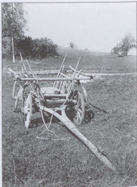
179. Szénaszállításra előkészített, négy nyírassal és két-két közzel felszerelt szekér. Jegenye (Kolozs vm.), 1991
