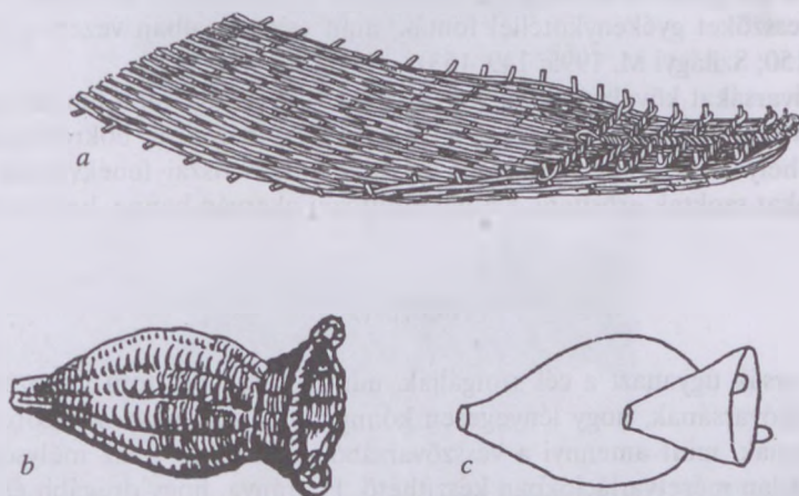
29. ábra. Egyszerű vesszővarsák: a) bocskorvarsa vagy magyar csuklyavarsa, Domokos (Szolnok-Doboka vm.); b) csíkvarsa, Közép-Tisza vidéke; c) csíkvarsa szerkezeti rajza
