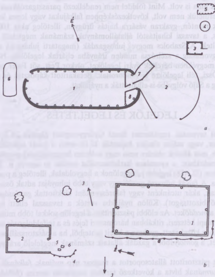
152. ábra. Juhász szállások elrendezési vázlata: a) 1. hodály, 2. karám, 3. kunyhó, 4-5. tyúkól, 6. nádrakás, 7. esztrenga, 8. szokató, Hajdúszoboszló (Hajdú vm.); b) 1. akol, 2. kolyiba, 3. csapás, 4. gát, 5. tűzhely, 6. patka, Váraszó (Heves vm.)
