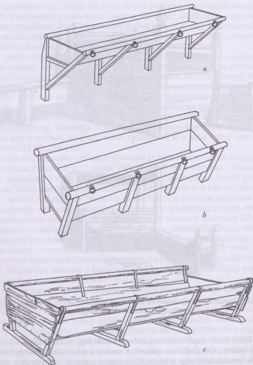
148. ábra. Jászolformák (1950 körül): a ) félszerjászol; b ) arcaljászol, Kismarja (Bihar vm.); c ) nyári jászol, Átány (Heves vm.)
