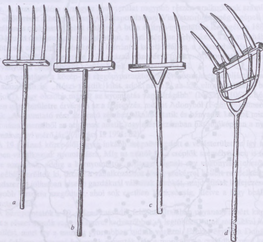
88. ábra. Törekhányó villák: a) Nagyjécsa (Torontál vm.); b) Sárpilis (Tolna vm.); c) Csenger (Szatmár vm.); d) Matolcs (Szatmár vm.)
