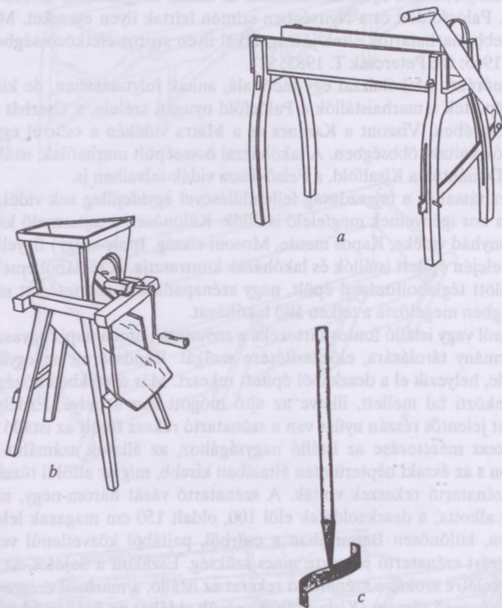
149. ábra. A takarmánykészítés eszközei: a) szecskavágó; b) hajtós répavágó (1950-es évek), Átány (Heves vm.); c) kézi répavágó, eselő , répa-s (1900 körül) Szentes (Csongrád vm.)
