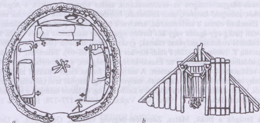
50. ábra. Erdőmunkások kunyhói: a) kerek kunyhó alaprajza, Répáshuta (Borsod vm.); b) jármás kunyhó rekonstrukciós rajza, Répáshuta (Borsod vm.)
