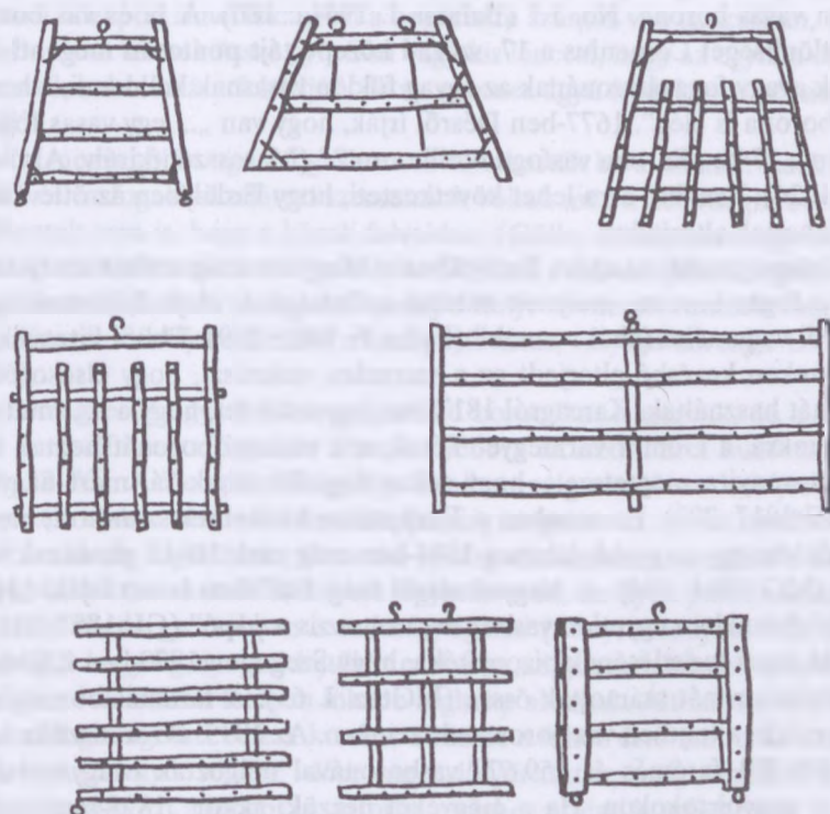
82. ábra. A favásas boronák főbb formái a Kárpát-medencében
