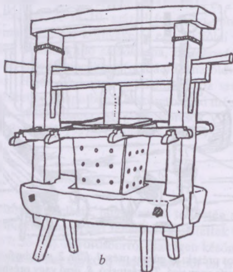
130. ábra. Erdélyi prések: a) medveprés: 1. medve, 2. köldök, 3. sróf, 4. orsó, 5. hajtórúd, 6. járom, 7. pap, 8. kas, 9. fák, 10. hátsó medve, 11. sajtókő, 12. kötés, 13-14. talp, Nagyenyed vidéke (Alsó-Fehér vm.); b) ékekkel működő prés, Váralmás (Kolozs vm.)
