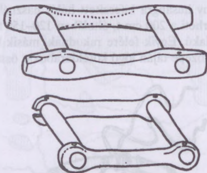
192. ábra. Zsákhordó keretek ( molnárlábak ) liszteszsák szájának széttárására és emelésére a malomban (1950-es évek), Kalotaszeg (Kolozs vm.)
