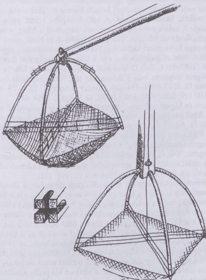
35. ábra. Örös emelőháló (csempely), Hernádbúd (Abaúj-Torna vm.)
