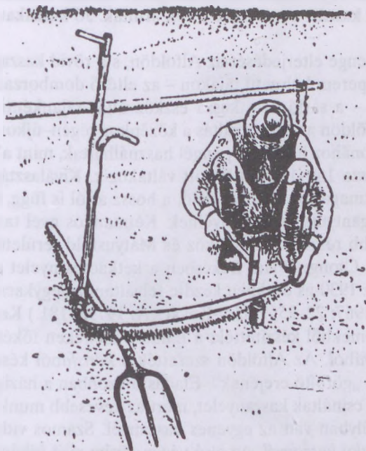
54. ábra. Nyélen fennhagyott kasza kalapálása, Dévaványa (Jász-Nagykun-Szolnok vm.)
