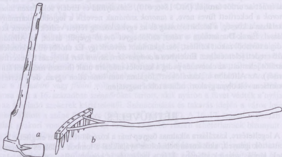
51. ábra. Rétművelési eszközök: a) irtókapa, Patca (Somogy vm.); b) talajgereblye, Gégény (Szabolcs vm.)
