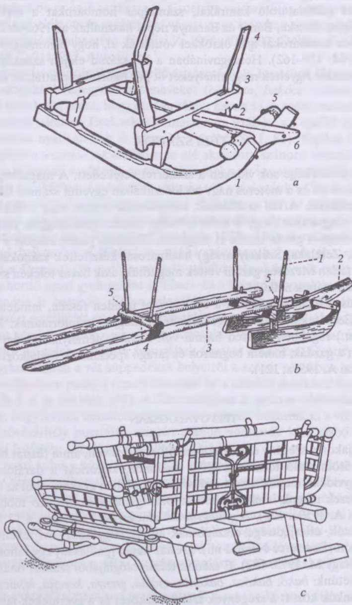
200. ábra. Téli szánok: a) marhaszán (1949 körül). Részei: 1. talp, 2. lába, 3. párna, 4. rókonca, 5. orsó, 6. oroc, Bogdánfalva (Moldva); b) nyoszolyás szán (1940 körül). Részei: 1. rókonca, 2. orcok, 3. nyoszolya, 4. keresztfa, 5. faszeg, Fenyéd (Udvarhely vm.); c) saroglyás lószán személyszállításra (1940 körül), Szentgál (Veszprém vm.)
