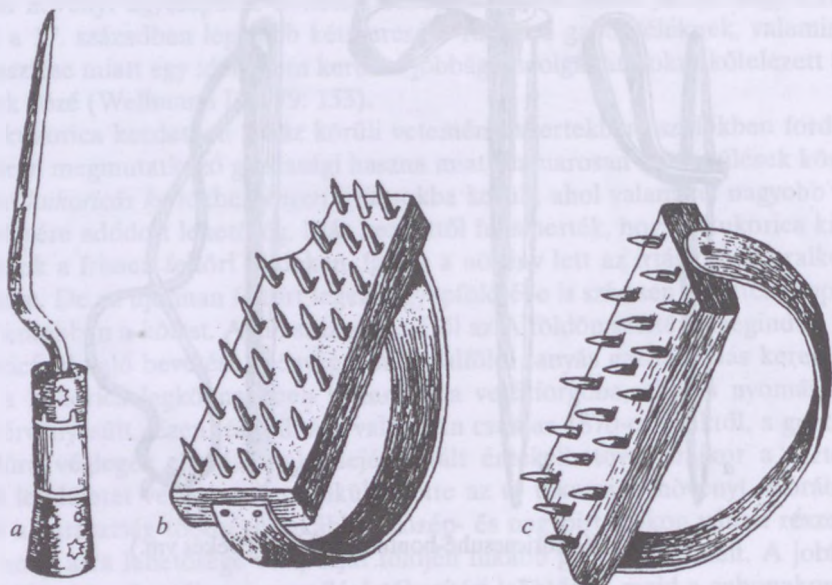
99. ábra. Kukoricamorzsoló eszközök: a) kukoricaszurkáló, Alföld; b–c) kukoricadörzsölők, Székelymuzsna (Udvarhely vm.)
