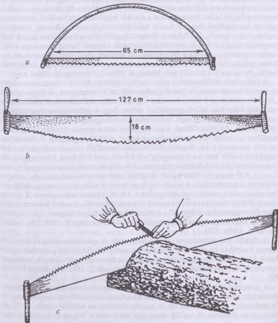
47. ábra. Fűrészek: a) cserfűrész; b) karajfűrész, Fülekpilis (Nógrád vm.); c) fűrész élesítése reszelővel
