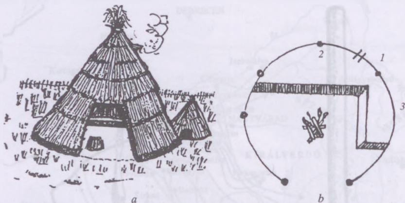
170. ábra. Kanászkunyhó makkos erdőben: a) előlnézete; b) alaprajza: 1. füstlyuk, 2. fekvő földpad, 3. ülő földpad (Somogy vm.)
