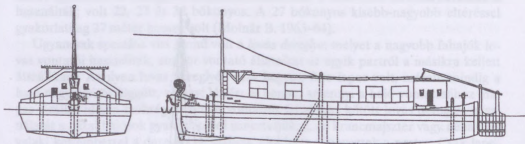
210. ábra. Tiszai bögőshajó kereszt- és hosszmeteszet rajza (19. század vége). Rekonstrukció, Deszk (Torontál vm.)
