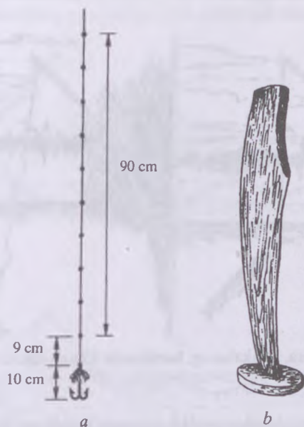
40. ábra. Puttyogató: a) a puttyogató zsinór szerkezete, Tiszaörvény (Heves vm.); b) kuttyogató, Algyő (Csongrád vm.)
