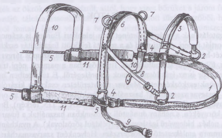
204. ábra. Igáshám lóra. Részai: 1. húzója, 2. vállkarika, 3. vállszíj, 4. csűrök, 5. estráng, 6. marszój, 7. gyeplőkarika, 8. segédszíj, 9. hasló, 10. hátszíj, 11. hámtáska (1920-as évek), Debrecen (Hajdú vm.)
