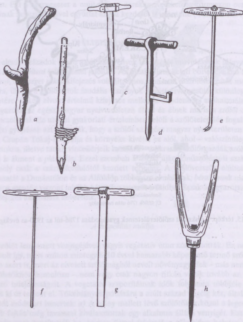
122. ábra. Szőlőültető fűrók: a ) természetes faágból, lépővel, Gyöngyösesorosi (Heves vm.); b ) kitáng természetes faágból, vesszőfonatos lépővel, Lujzikalagor (Moldva, Románia); c ) T alakú ültetőfűró, beékelt, esztergált fogóval, Cegléd (Pest-Pilis-Solt-Kiskun vm.); d ) T alakú ültetőfűró kovácsoltvas szárral, lépővel és fa fogóval, Visonta (Heves vm.); e ) körmos fűró, Kecel (Pest-Pilis-Solt-Kiskun vm.); f – g ) T alakú ültetőfűró és szorító, Kecel (Pest-Pilis-Solt-Kiskun vm.); h ) Y alakú ültetőfűró, Dunaföldvár (Tolna vm.)
