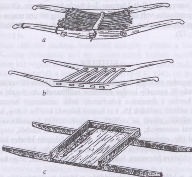
190. ábra. Teherhordó saroglyák: a) cserény (1950 körül), Átány (Heves vm.); b) saroglya (1950 körül), Átány (Heves vm.); c) ganéhordó saraglya (1940), Kolozsvár-Hóstát (Kolozs vm.)
