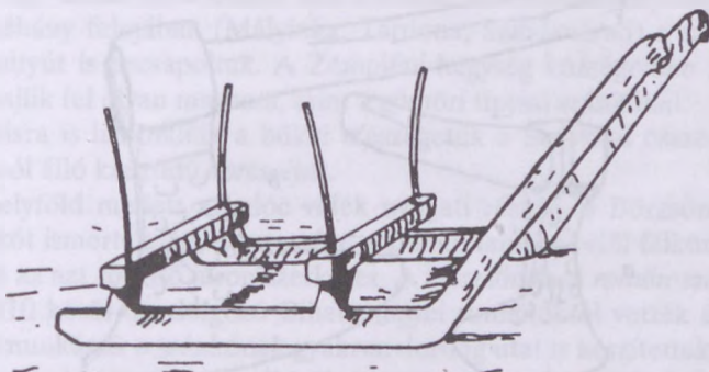
48. ábra. Erdei gyalogszánkó ölfá szállításához, Csermosnya-völgy (Gömör és Kishont vm.)
