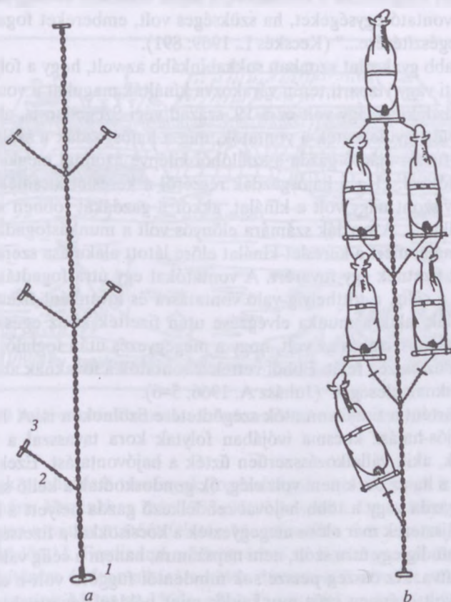
212. ábra. Vontatólovak befogása: a) vontatórúd. Részei: 1. a rúd drumója, 2. pajzer, 3. pajzerpecsek; b) a lovak befogásának sémája (19. sz. második fele), Deszk (Torontál vm.)
