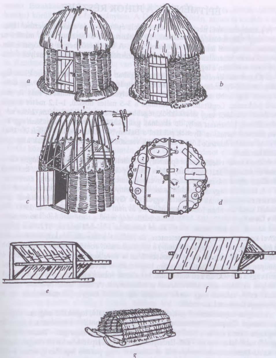
158. ábra. Juhászkunyhók (esztenák) a legelőn: a) ellipszis alaprajzú esztena; b) kör alaprajzú esztena; c) az esztena szerkezete: 1. szelemen, 2. oldalágas, 3. középpágas, 4. káva; d) az esztena belső berendezése: 1. láda, 2. cseber, 3. krinta, 4. deberke, 5. sajtprés, 6. sajtpolc, 7. kisszék, 8. tűzhely, 9. középpágas, 10. üstfa, 11. szék, 12. tűzrevaló, 13. vizesedény, 14. galáták, 15. oldalágas, 16. kereszttrúd, 17. ajtó, Bálványosvára (Szolnok-Doboka vm.). Hordozható juhászkunyhók: e) féleresztes sárik, Körös (Gömör és Kishont vm.); f) nyereggetős koliba, Cakó (Gömör vm.); g) vontatható kaliba (1940-es évek eleje), Sztána (Kolozs vm.)
