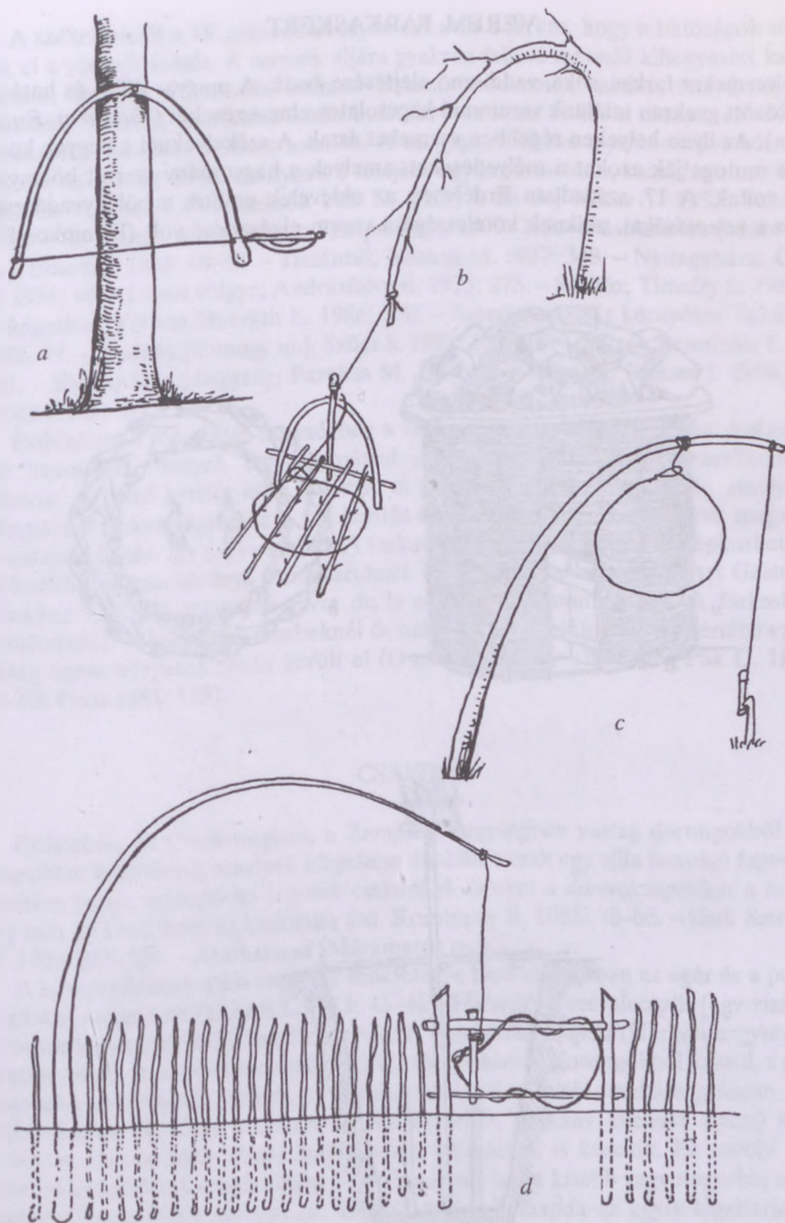
11. ábra. Rántóhurkok: a) pruglo típusú rántóhurkok, Torockó (Torda-Aranyos vm.); b) talpkioldású felrántóhurkok, Felsőrcsecsin (Moldva); c) magyar csikkentő őz fogásához, Domokos (Szolnok-Doboka vm.) d) csikle vízimadarak fogásához, Kopács (Baranya vm.)
