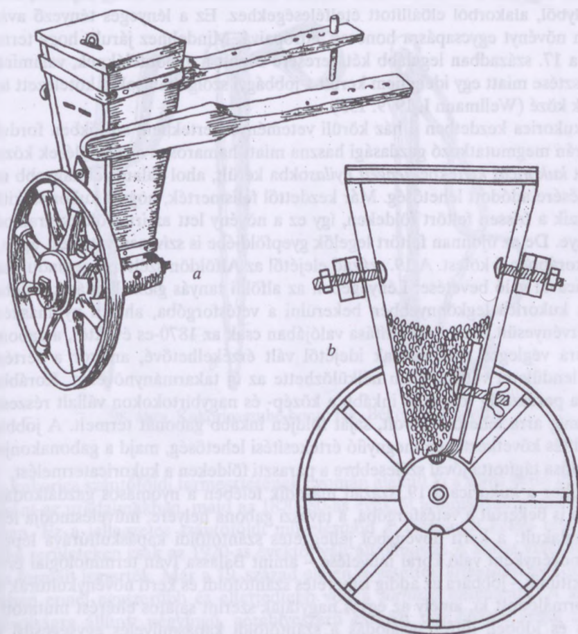
97. ábra. Kukoricavető eszközök: a) ekére szerelhető kukoricapergető; b) a pergető keresztmetszete, Hódmezővásárhely (Csongrád vm.)
