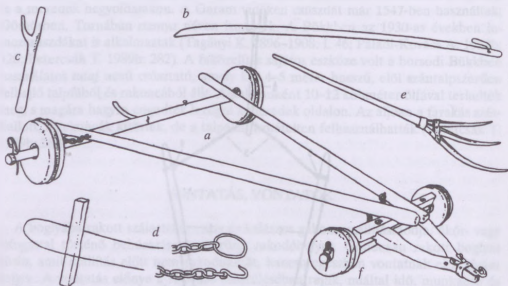
198. ábra. Kerekcs vontató és tartozékai (1950 körül): a) vontatókocsi; b) kisirud vagy rudasfa; c) inas; d) húzatólánc; e) favilla, Hódmezővásárhely (Csongrád vm.)
