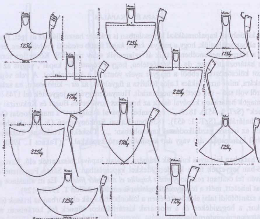
71. ábra. Mecenzéfen kovácsolt magyar kapaformák
