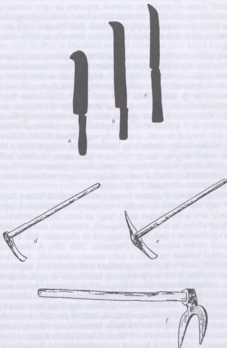
68. ábra. Az irtás eszközei: a–c ) irtókések (Vas vm.); d ) ortókapa, Nagyhuta (Abaúj-Torna vm.); e ) csákány, Nagyhuta (Abaúj-Torna vm.); f ) kétágú ágaskapa, Kishuta (Abaúj-Torna vm.)
