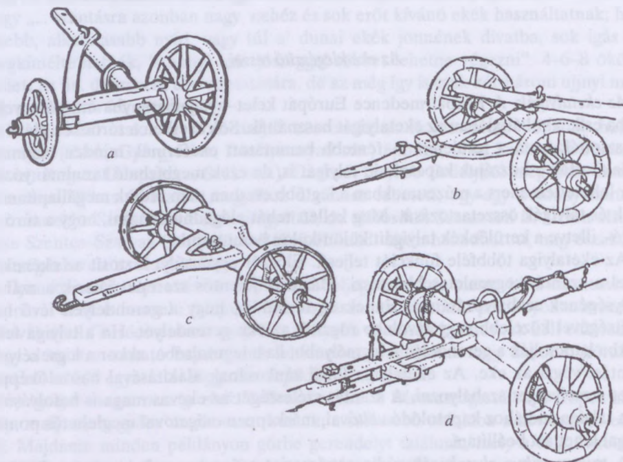
75. ábra. Eketaligák fa kerülőekéhez: a) bőr patinggal , Onyest (Moldva, Románia); vasfejű váltóekékhez: b) Ajton (Kolozs vm.); c) Katona (Kolozs vm.); d) Mezőköbőkút (Kolozs vm.)
