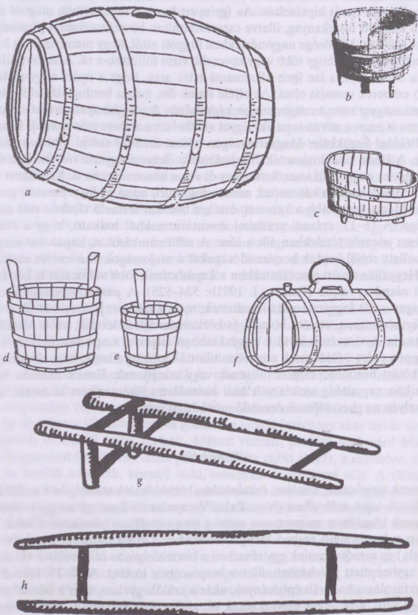
132. ábra. Pincegazdasági eszközök: a) boroshordó; b–c) hordótölcsérek (általános formák); d–e) finak és fertály, Tiszakécske (Pest-Pilis-Solt-Kiskun vm.); f) légely, Nagyenyed vidéke (Alsó-Fehér vm.); g) hordóhajtó csántér (általános forma); h) korcsolya vagy kúcsorja (általános forma)
