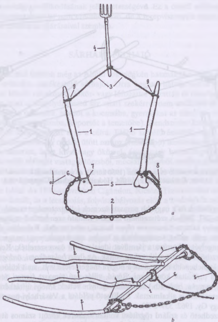
197. ábra. Vontatófák: a) régebbi fajta vontatófa (1940-es évek). Részei: 1. rúd, 2. talpalólánc, 3. istrangok, 4. akasztóvilla, 5. butykója, 6. kompósszeg, 7. perec, 8. kapacs, 9. az istrangok urka, Kolozsvár, Hóstát (Kolozs vm.); b) újabb fajta vontatószánka. Részei: 1. előfa vagy járna, 2. talpak vagy villásrúdok, 3. köze, szárnyak vagy csúsztatók, 4. slófos szegek, 5. talpalólánc, 6. csatláslánc, Kolozsvár, Hóstát (Kolozs vm.)
