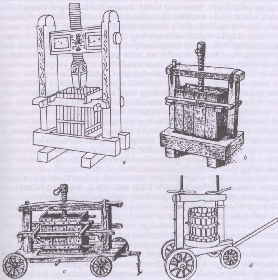
131. ábra. Középsős prések vagy sajtók: a) alulhajtós sajtó, Soltvadkert (Pest-Pilis-Solt-Kiskun vm.); b) felülhajtós sajtó, Borsodgeszt (Borsod vm.); c) középsős, felülhajtós, kerekes sajtó, Kecskemét (Pest-Pilis-Solt-Kiskun vm.); d) állóorsós, kerekes sajtó, Kiskunhalas (Pest-Pilis-Solt-Kiskun vm.)
