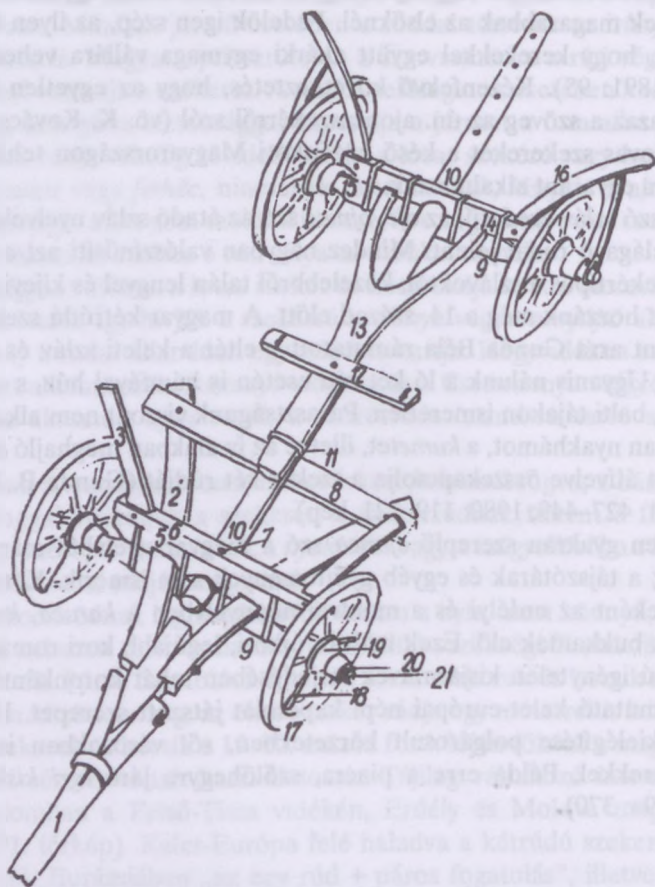
202. ábra. A hegyközi szekér szerkezete (1950-es évek): 1. rúd, 2. ágas, 3. rakonca, 4. tengely, 5. simely, 6. fergettyű, 7. derékszög, 8. juha, 9. cugpánt, 10. nyújtó, 11. nyújtókarika, 12. féktartó, 13. hátsóágas, 14. simely, 15. ánstok, 16. löcs, 17. keréktalp, 18. küllő, 19. agy, 20. tengelyvégszeg, 21. persely, Pusztafalu (Abaúj-Torna vm.)
