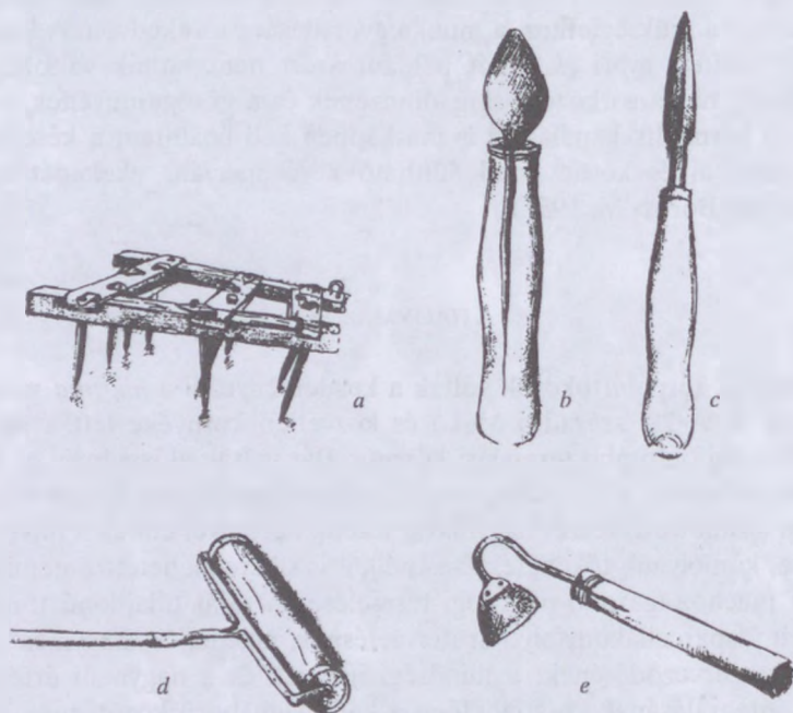
111. ábra. Makói hagymások eszközei: a) favázás, kézi kisfogas ; b) régi típusú hagymaásó; c) az 1950-es években elterjedt hagymaásó; d) henger; e) apróhagyma kaparó
