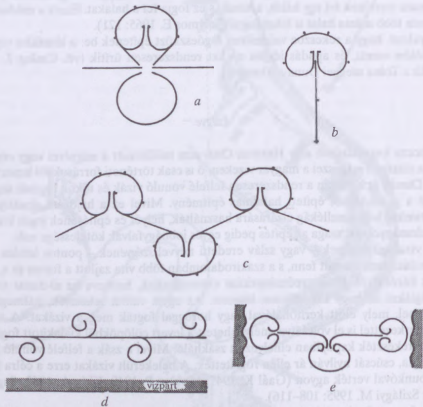
27. ábra. Vejszék: a) udvaros, kétszárnyas vagy magyar vejsze, Tápé (Csongrád vm.); b) középlészás vejsze, Tápé (Csongrád vm.); c) kétszárnylészás vagy rácvejsze, Mezősegi tavak (Erdély); d) spirálvejsze, Szentés (Csongrád vm.); e) középlészás és kétszárnylészás vejszék kombinációja, Közép-Tisza-vidék
