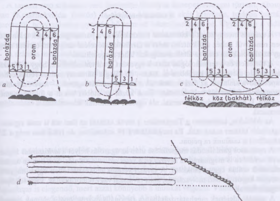
78. ábra. A kerülőekes szántás barázdavonal menete: a) összeszántás; b) szétszántás; c) bakhátas szántás; d) a váltóekes szántás barázdavonal-menete
