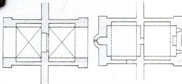
Црѡеж основе њорше, ѡриземље и сѡрајѡ – реконструкција
