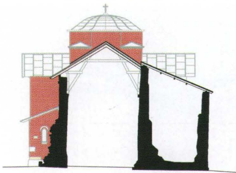
Манастир Бањска, њоречни и њодужни ѡресек
