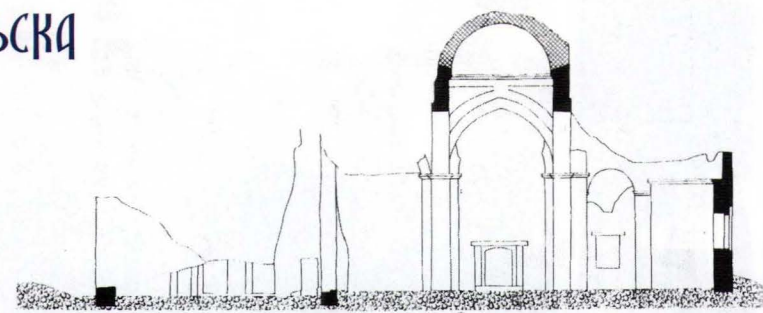
Пресек и основа цркве Св. Стефана
