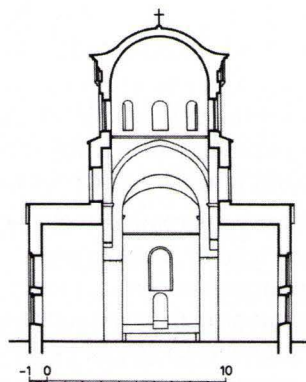
Појречни пресек кроз куйолу
