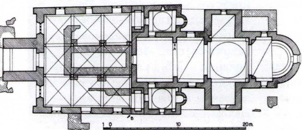
Подужни пресек и основа цркве Вазнесења Христјовој
