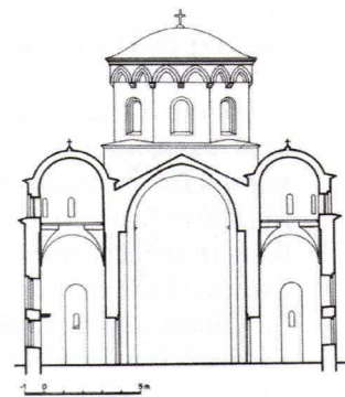
Појречни пресек кроз иријрају и бочне капеле
