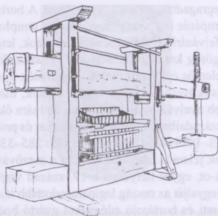
212. ábra. Kőhúzás bálvánsajtó. Tolcsva (Zemplén vm.)
