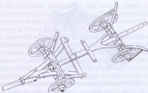
215. ábra. Szekér alváza első és hátsó ágassal, nyújtóval, rakoncákkal. Hegyköz (Abaúj-Torna vm.)
