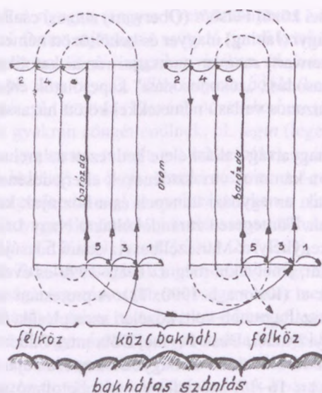
16. ábra. A bakhátas szántás sematikus rajza
