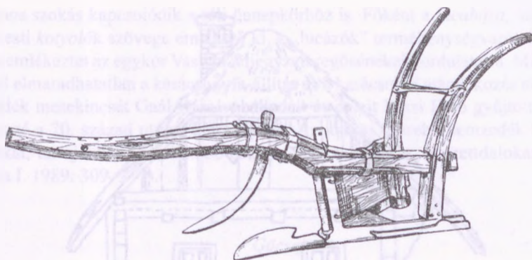
23. ábra. Görbe gerendelyű faeke. Kúpfalva (Vas vm.)
