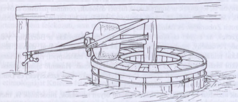
170. ábra. Kőtelesmester kendermorzsolója. Vác (Pest-Pilis-Solt-Kiskun vm.)
