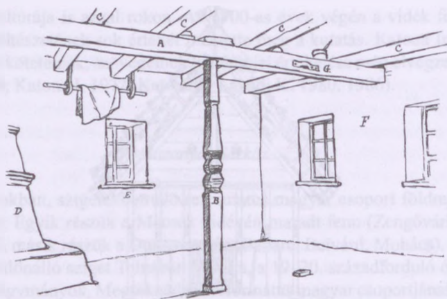
104. ábra. Mestergerenda ( ideg ) és idegágas . Szentlászló (Verőce vm.)
