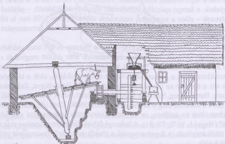
61. ábra. Taposómalom szerkezete. Bakonypéterd (Veszprém vm.) 1930-as évek
