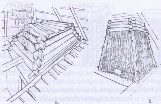
225. ábra. a) Vakkémény, füstfogó a padlásán. Nagydoba (Szilágyság vm.), b) Kezdetleges kémény, belül sárral tapasztva. Désháza (Szilágyság vm.)
