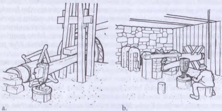
238. ábra. a) Verő. Kapahámor farkkalapácsa. b) Kapaverő munkában. Torockó (Torda-Aranyos vm.)
