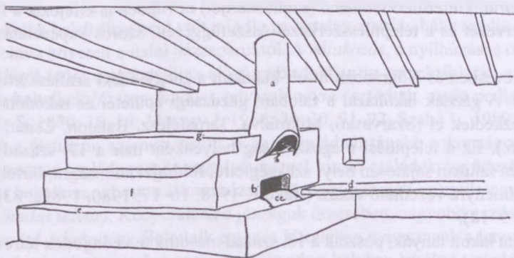
174. ábra. Kürtös kemence. Parád (Heves vm.)
