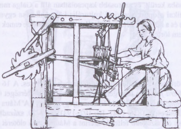
185. ábra. Palóc szátva, Galgamácsa (Pest-Pilis-Solt-Kiskun vm.)
