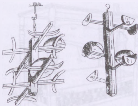
37. ábra. Kenyértartó rács. Velem (Vas vm.) 20. század eleje
