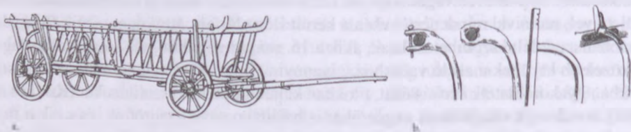
263. ábra. a) Hordólajtorjás székér. b) Lőcsők: sutalócs , bágyi lőcs, ágas lőcs (Udvarhely vm.)
