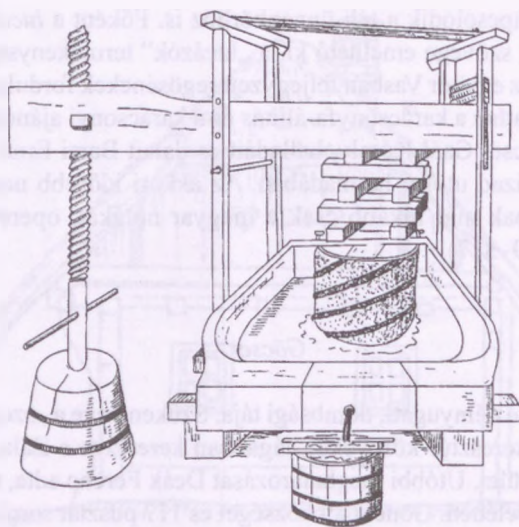
26. ábra. Gúzsos prés. Cserfő (Zala vm.) 1940-es évek
