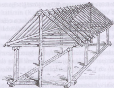
58. ábra. Sövényház váza. Balatonmellék
