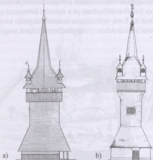
122. ábra. Református harangtorony homlokzata: a) Nyírbátor, b) Zsurk (Szabolcs vm.)
