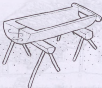
279. ábra. Tekenyő szőlőtaposáshoz. Lészped (Moldva)
