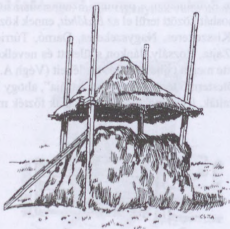
109. ábra. Abara. Szénatároló csúsztható fedéllel. Beregi Tiszahát
