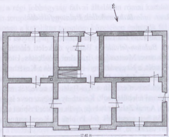
68. ábra. Kossuth Lajos kúriájának alaprajza. Tinnye (Pest-Pilis-Solt-Kiskun vm.)
