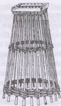
132. ábra. Vesszőtapogató, halászeszköz. Békés (Békés vm.)
