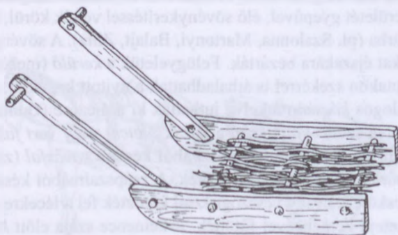
198. ábra. Körcsolya köcsüsztatáshoz. Bélapátfalva (Borsod vm.)
