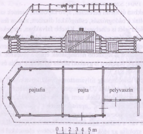
31. ábra. Sokszögű csűr. Külsősárd (Zala vm.)
