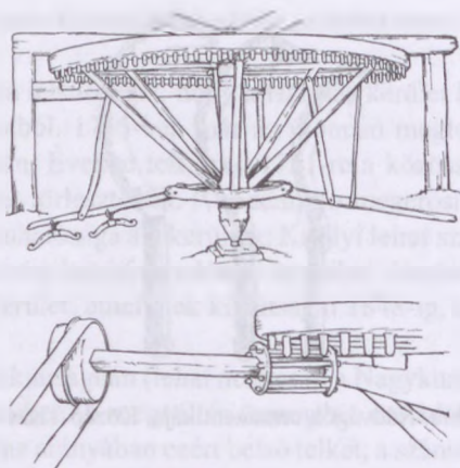
131. ábra. Kunsági olajütő keringője és orsója . Kunmadaras (Jász-Nagykun-Szolnok vm.)
