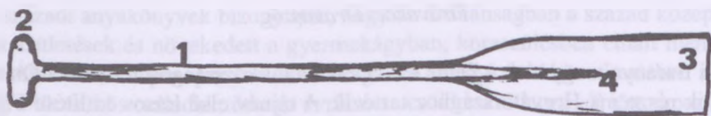
99. ábra. Dali evező részei: 1. szár, 2. bodé, 3. lap, 4. ér. Kopács (Baranya vm.)
