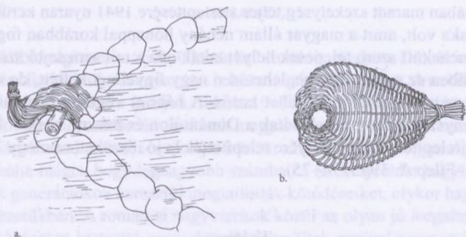
285. ábra. a) Sejp, „bocskorvarsa” kőből épített gát csorgóján, b) közönséges vesszővarsa. Andrásfalva (Bukovina)
