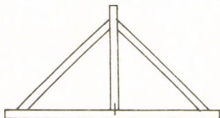
egyszeres függesztőmű
