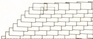
fekvő téglányfedés
