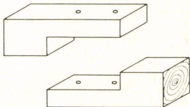
egyenes lapolás
