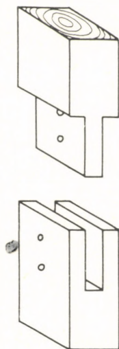
ollós csapolás
