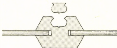
műanyag szalagos, szorítóléces üvegezés
