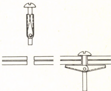
szétnyíló vállú lemezcavar
