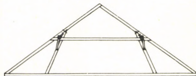
b) két dűltszékes fedélszék
