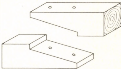
ferde lapolás
