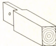
csapolás
