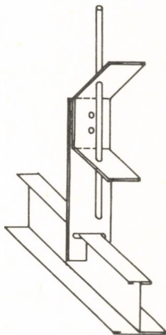
állítható felfüggesztés
