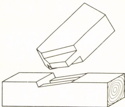
b) egyszeres ferde csapos beeresztés
