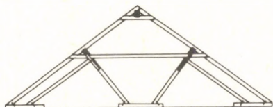
bakdúcos fedélszék
