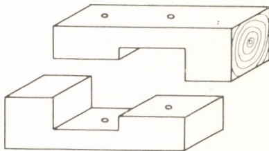
fogas lapolás
