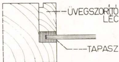
üvegszorító lécz
