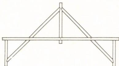
egyesített függesztő- és feszítőmű
