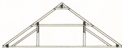
a) két állószékes fedélszék
