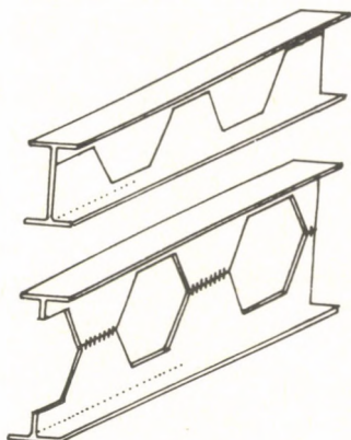
takaréküreges tartó
