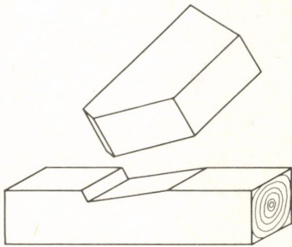
a) egyszeres ferde beeresztés
