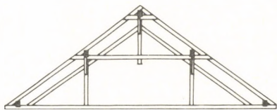
háromszékes fedélszék
