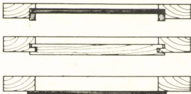
táblázatos faburkolat
