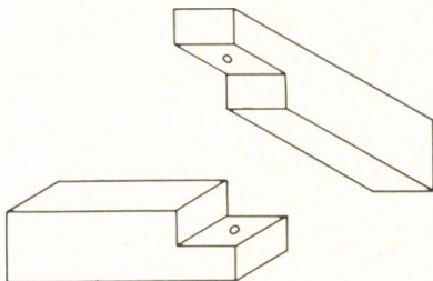
saroklapolás
