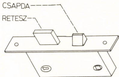
bevéő vasalat
