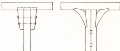
hónaljfa
