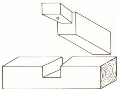
fecskefarkkötés
