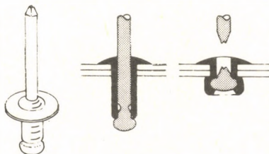
húzószegecs
