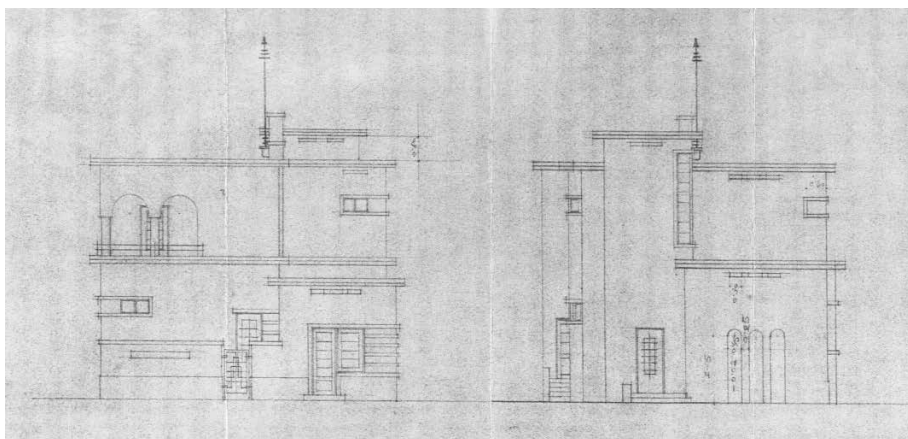
1. kép Dr. Székely Gyula és Steiner Éva házának homlokzati rajza
