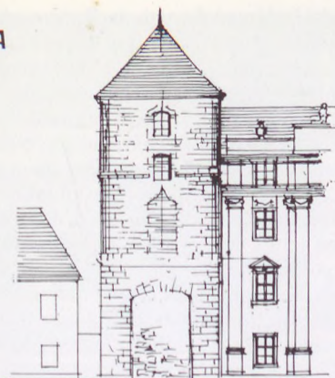
A torony a XVIII-XIX. században (A) (Sedlmayr János rekonstrukciója) és 1934 után (B) (Lux Kálmán építész tervei szerint)
