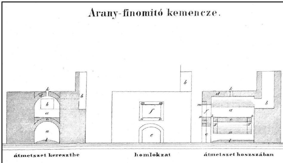
1. ábra. A nagybányai aranyfinomító kemence felépítése.
