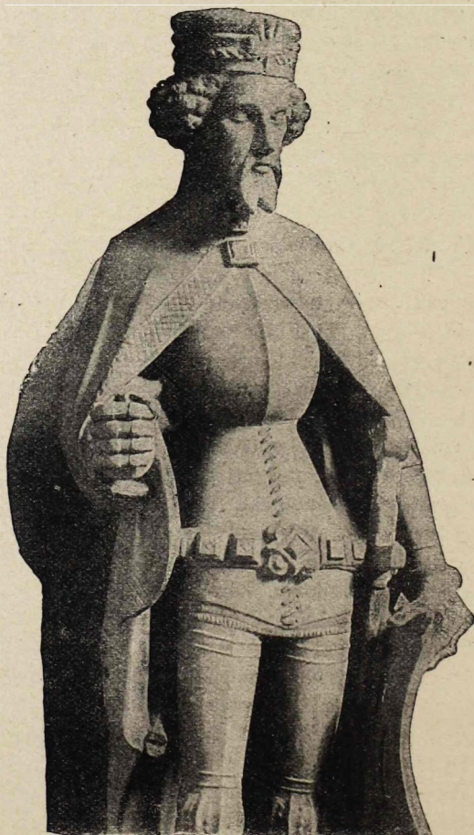
IV. Károly német-római császár.
