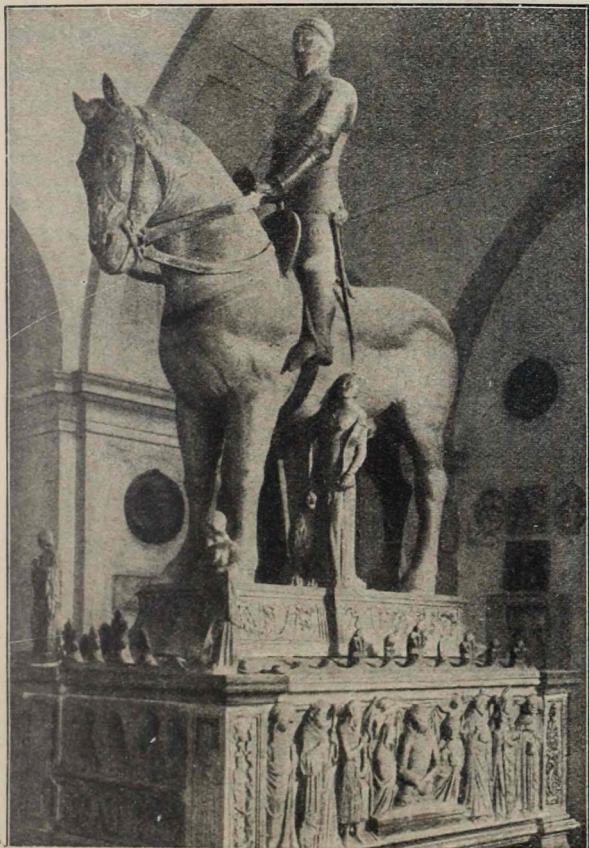
Visconti Barbano szobra.
