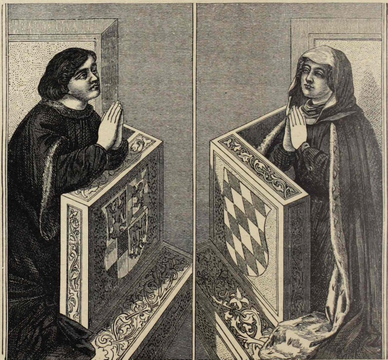
Frigyes brandenburgi választófejedelem és felesége, Erzsébet.
