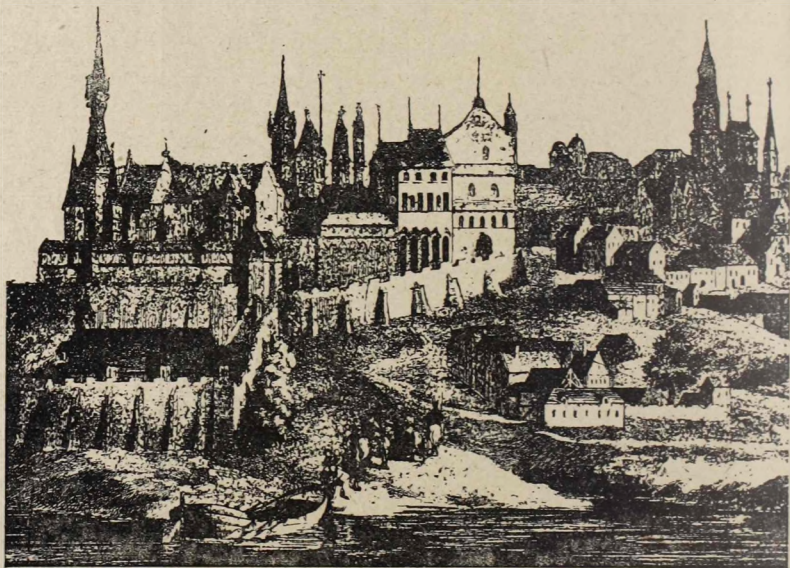
Budavára Mátyás király idejében.
