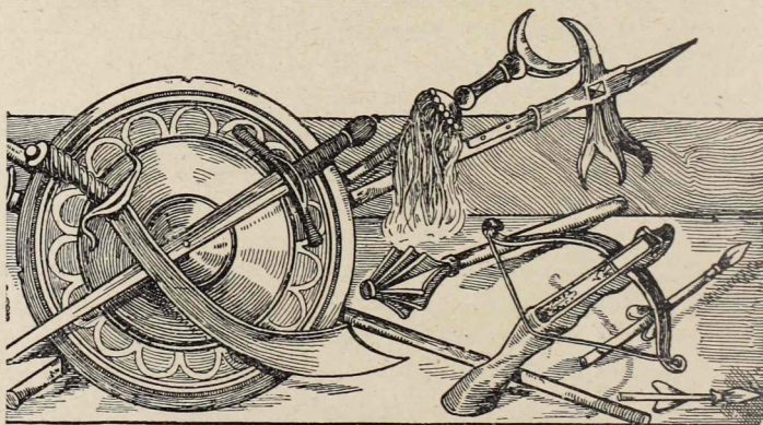
Nagy Lajos korában használt magyar és török jegyverek.
