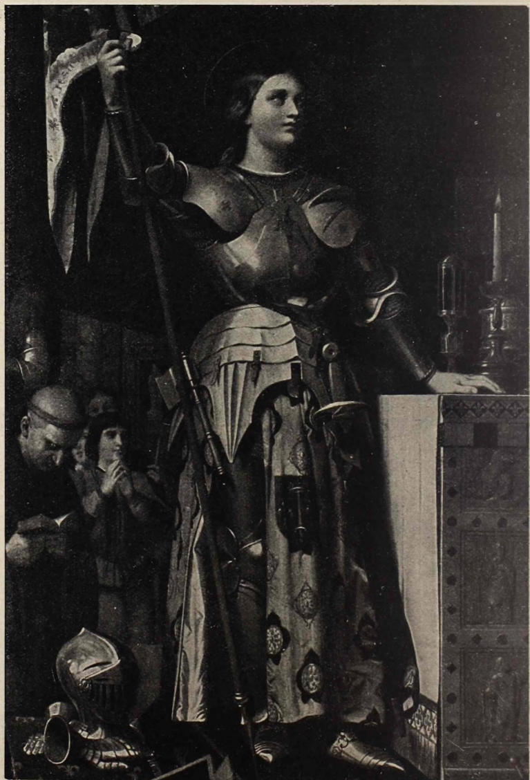
Jeanne d'Arc, az Orleánsi szűz. Látományai folytán rendithetetlenül meg volt győződve arról, hogy isteni küldetése van hazájának az angol uralom alól való felszabadítására. Rajongó lelkesedése áthatja a francia csapatokat, amelyekkel egymás után aratja győzelmeit az angolok fölött. Compiègne mellett az angolok elfogják. Boszorkánysággal vádolva egyházi port indítanak ellene s máglyán égetik el. Később szentté avatták s a franciák nemzeti hős gyanánt tisztelik ma is.
