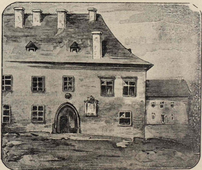
Mátyás király emléktáblával megjelölt szülőháza Kolozsvárott.
