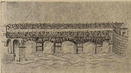
Trajánusz császár dunai hidjának rajza. A császár római diadaloszlopán lévő dombormű.
