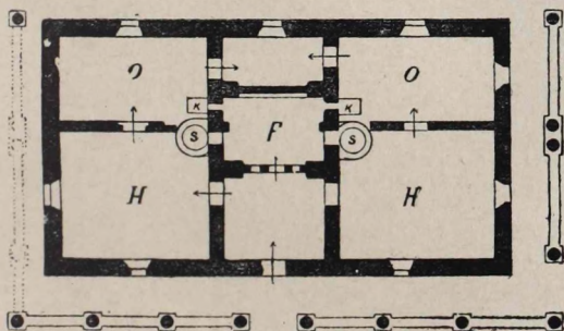
Nemesi kúria, Kemecse (Szabolcs megye). F = fűstház; O, H = szobák.
