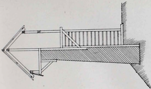
Középkori védőfolyosó kereszt- metszete. (Könyöki József; Középkori várak e. műből.)
