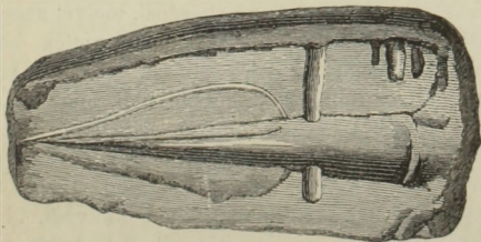
Bronz-lándzsafej öntésére szolgáló félminta homokkőből. Fugyi-vásárhelyi lelet. \frac{1}{2} nsg.
