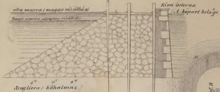
(A csövek el közepi homlokzata / Profilo medio della Palafitta
