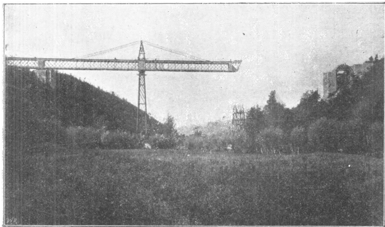
VIADOTTO OLONA. A nagy híd áttolása egy darabban.
