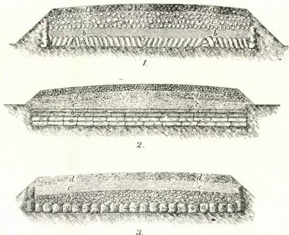
1—3. Rajnamenti kavicsolt római utak (Glarea viam sternere)
