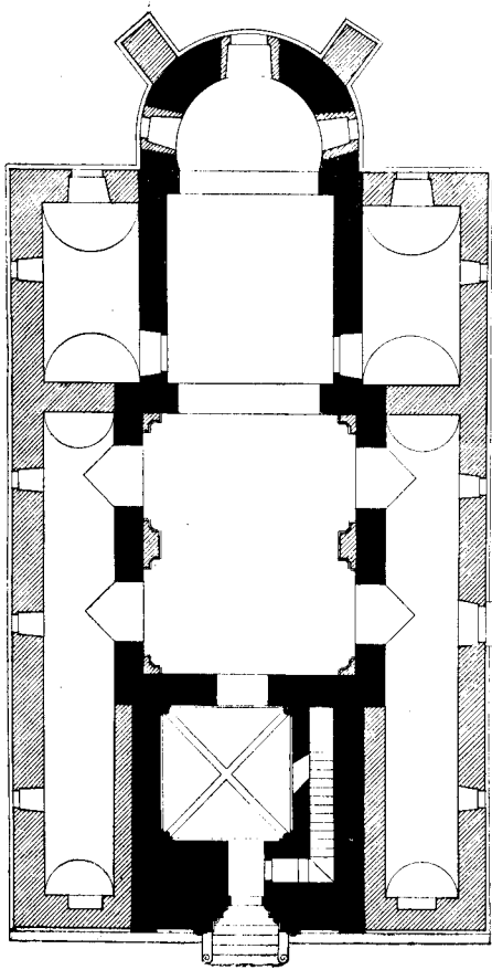
13. Földszinti alaprajz.
