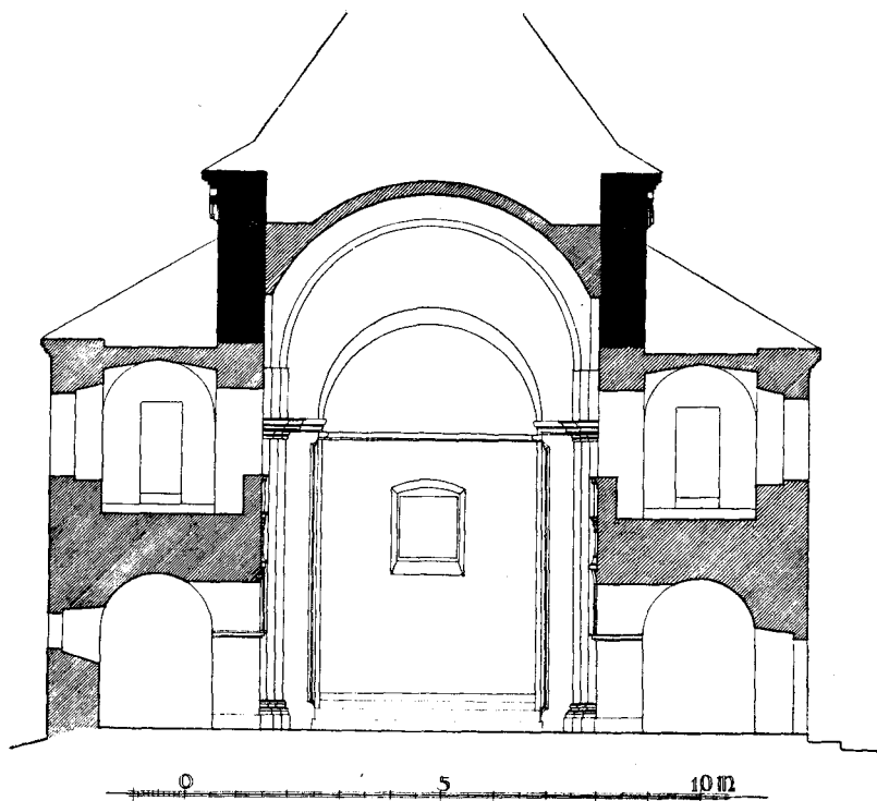
12. A templom keresztmetszete.
