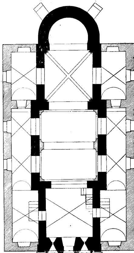
14. Emeleti alaprajz.
