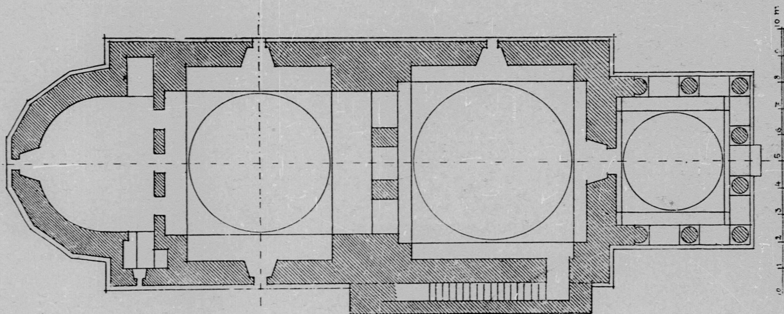
Biserica din Vădeni (Gorj) Fig. 232. — Planul orizontal
