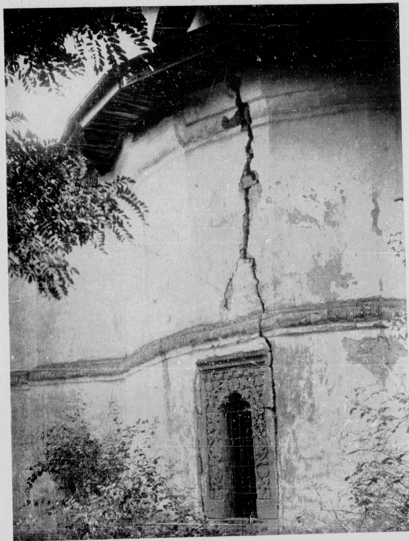
Fig. 943. — Detaliu de fațadă
