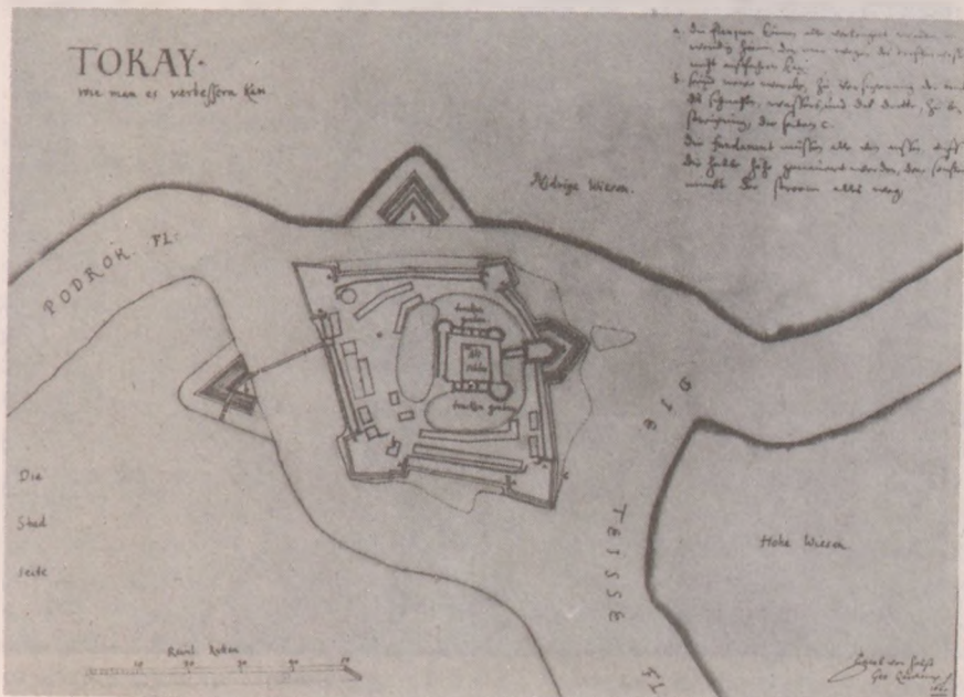
„Tokaj, ahogyan jobbítható”, Jacob von Holst alaprajza, 1660.
