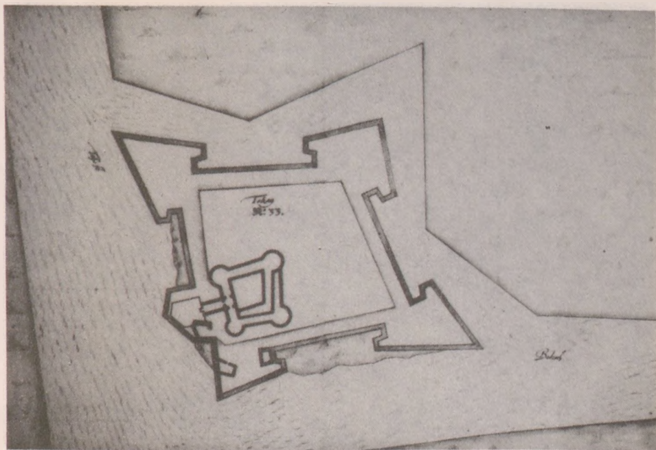
Tokaj várának fülesbástyás alaprajza Poppendorf javaslata szerint, 1570 körül. Az osztrák Nemzeti Könyvtár kéziratárában.
