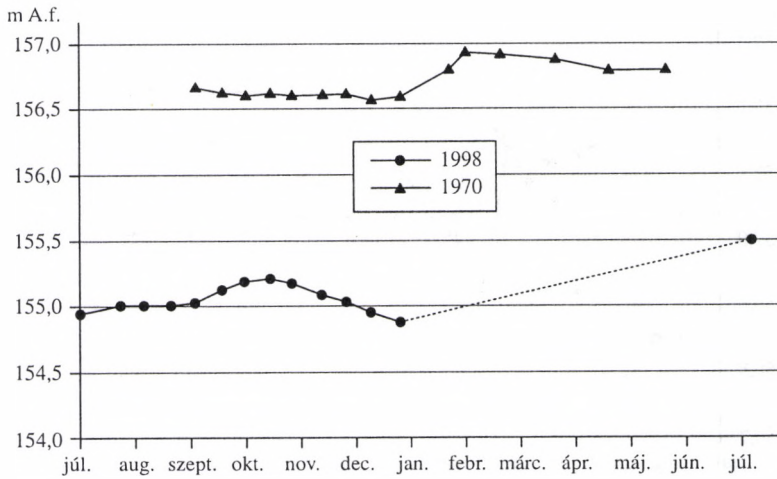
3.14. ábra. A Hadik kút vízállás-idősorai
