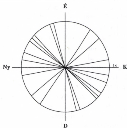
2.11. ábra. Az édesvízi mészkő litoklázisainak gyakoriság diagramja, Tánicsics Mihály utca
