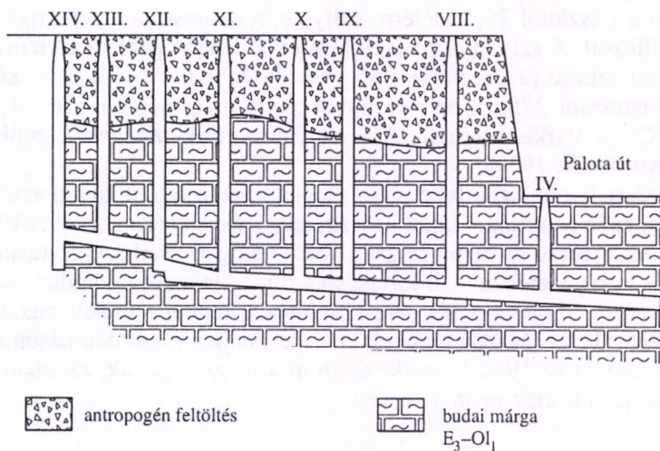
3.25. ábra. A víztelenítési mű alaprajza és metszete (HORUSITZKY F. nyomán)
