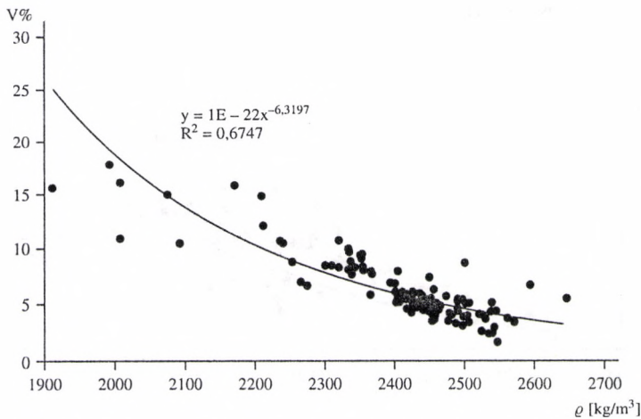
3.8. ábra. Az édesvízi mészkő testsűrűség látszólagos porozitásdiagramja
