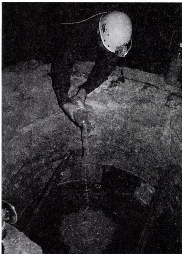
4. kép. Vízfestéses vizsgálat az áramlási viszonyok megállapítására (Czakó L. felvétele)
