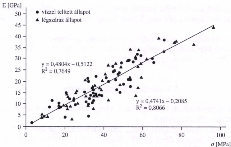
3.7. ábra. Az édesvízi mészkő nyomószilárdság-rugalmassági modulusdiagramja
