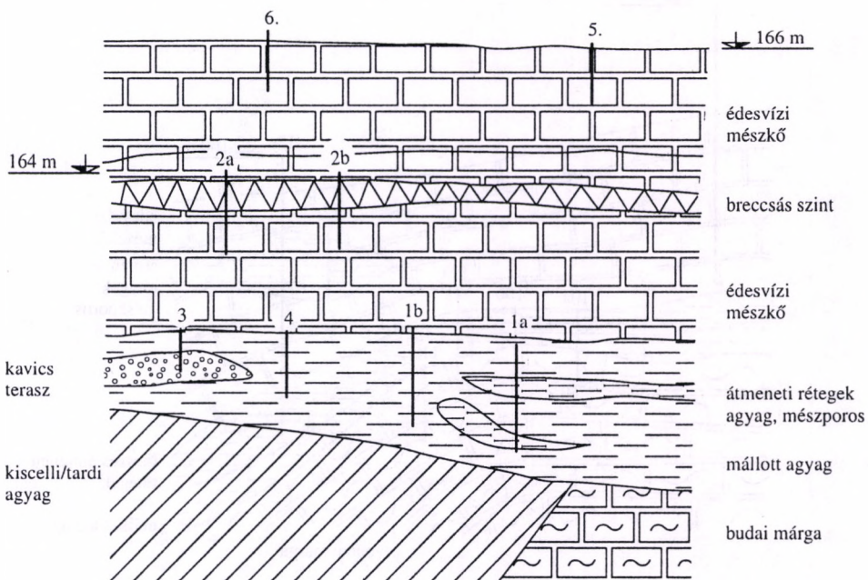
2.3. ábra. A budai Várhegy É-i részének szelvény-korrelációja (TÖRÖK et al. 1998 nyomán)
