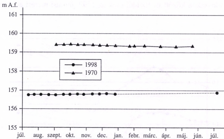
3.17. ábra. A Mérőórás kút vízállás-idősorai
