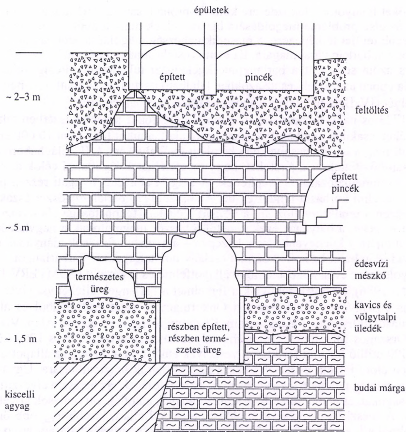
3.1. ábra. Pince- és üregrendszer típusszelvénye
