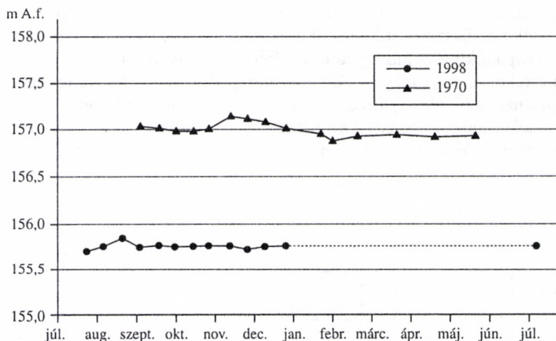
3.11. ábra. A Kávészó kút vízállás-idősorai
