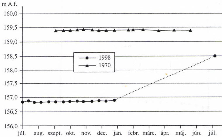
3.18. ábra. A Barlangos kút vízállás-idősorai
