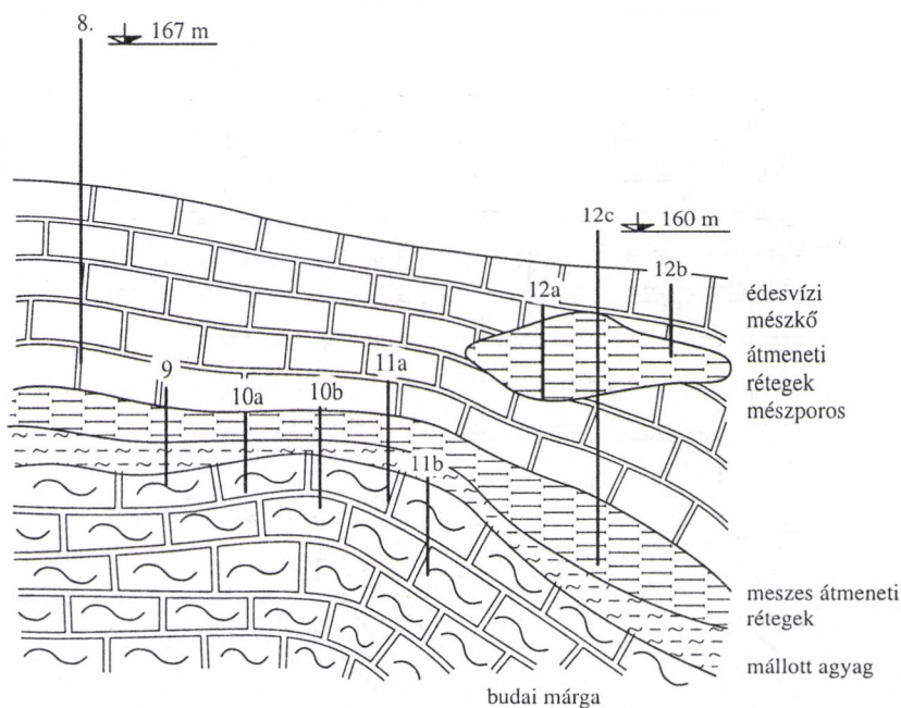
2.4. ábra. A budai Várhegy D-i részének szelvény-korrelációja (TÖRÖK et al. 1998 nyomán)
