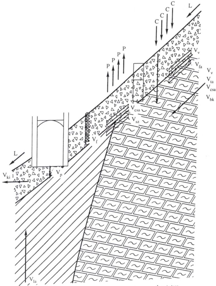
4.8. ábra. A vízmérleg elemei a Lejtőre vonatkoztatva
