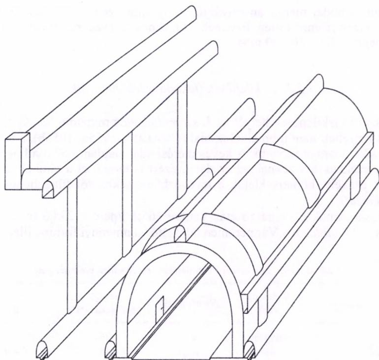
3.20. ábra. Az Alagút térbeli elhelyezkedése a víztelenítő vágatokkal
