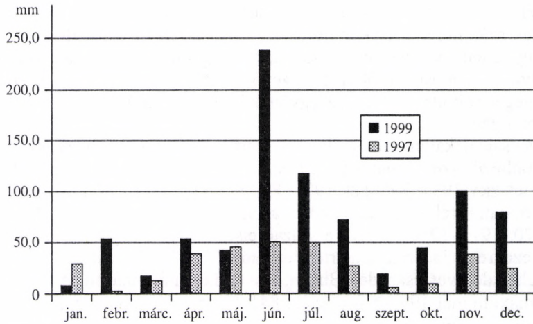
4.2. ábra. Havi csapadékatatok összehasonlítása 1997. és 1999.
