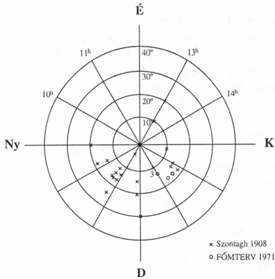
2.7. ábra. A budai márga dőlésiránya és dőlésszöge
