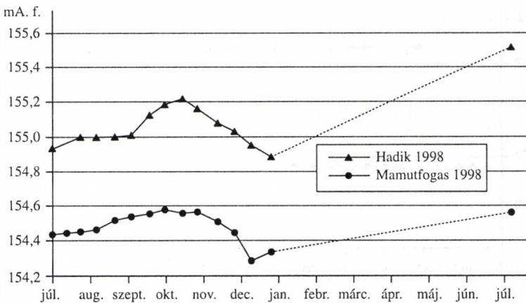
3.19. ábra. A Hadik- és a Mamutfogas kút vízállás-idősorainak összehasonlítása
