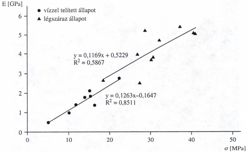
3.3. ábra. A budai márga nyomószilárdság-rugalmassági modulus diagramja
