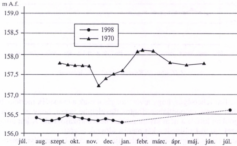
3.9. ábra. A Bőlényes kút vízállás-idősorai
