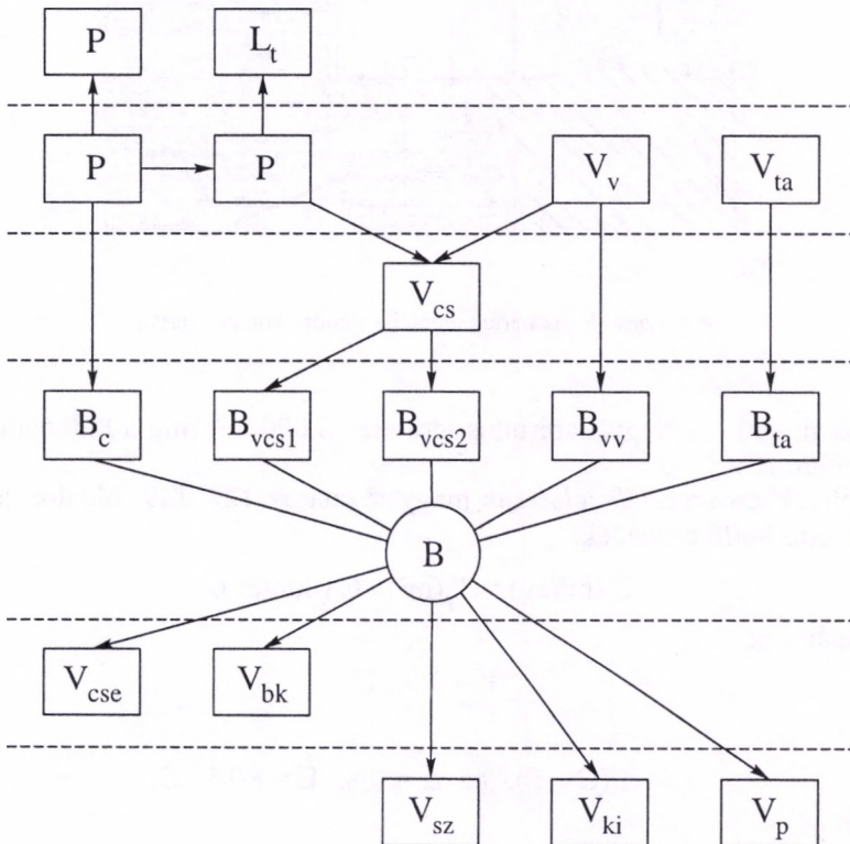
4.6. ábra. A vízmérlegszámítás folyamatábrája
