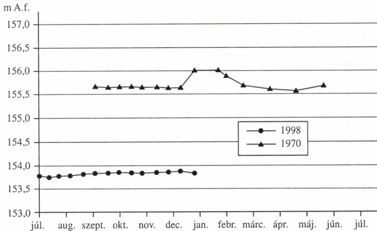
3.15. ábra. A Török kút vízállás-idősorai
