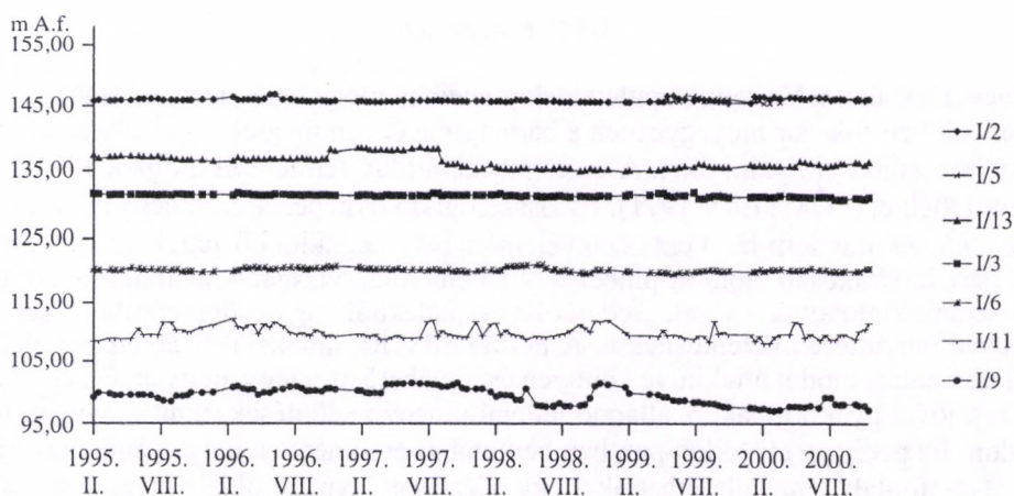
3.24. ábra. Talajvízszint-észlelő kutak adatsorainak összehasonlítása
