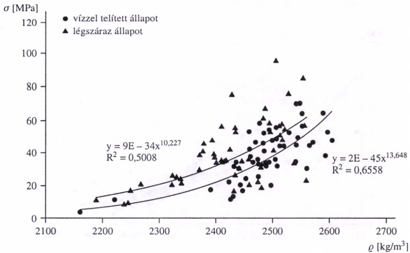
3.6. ábra. Az édesvízi mészkő testsűrűség-nyomószilárdság diagramja
