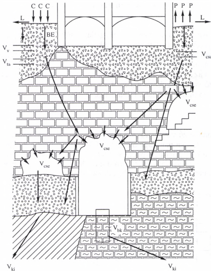
4.7. ábra. A vízmérleg elemei a Platóra vonatkoztatva
