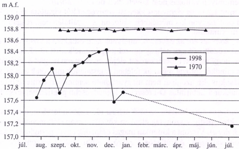
3.10. ábra. A Nagy kút vízállás-idősorai
