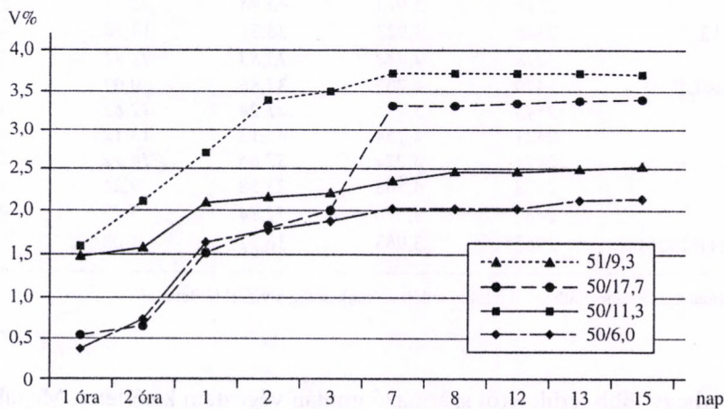
3.5. ábra. A budai márga vízfelvele
