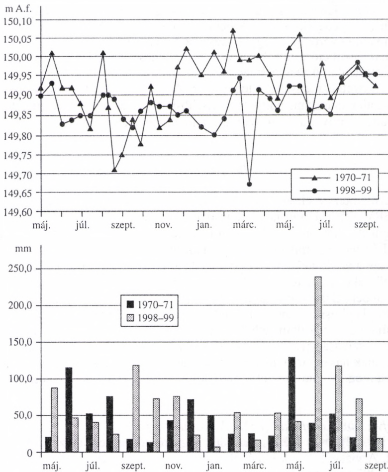
3.21. ábra. I/2. Fiáth János u. 2. Talajvízszint-észlelő kút adatsora
