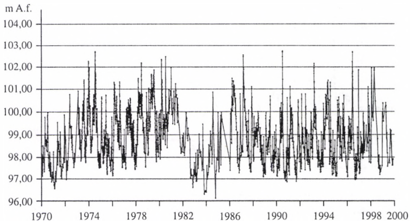
3.23. ábra. I./9. Bem rakpart 28. Talajvízszint-észlelő kút adatsora
