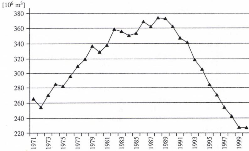
4.5. ábra. Budapest évi vízbetáplálása
