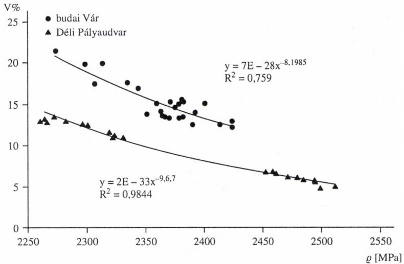
3.4. ábra. A budai márga testsűrűség-látszólagos porozitás diagramja
