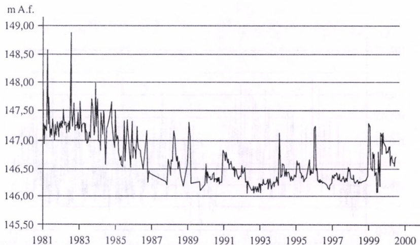
3.22. ábra. I/5. Lovas út 9. Talajvízszint-észlelő kút adatai
