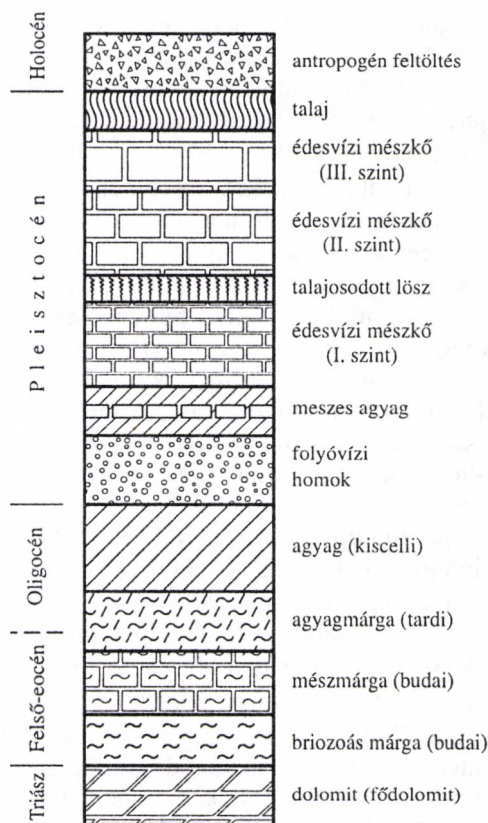
2.2. ábra. A budai Várhegy rétegsora (HORUSITZKY 1939 és TÖRÖK et al. 1988 nyomán; Ezek a kőzetjelölések érvényesek a további földtani ábrákon is)
