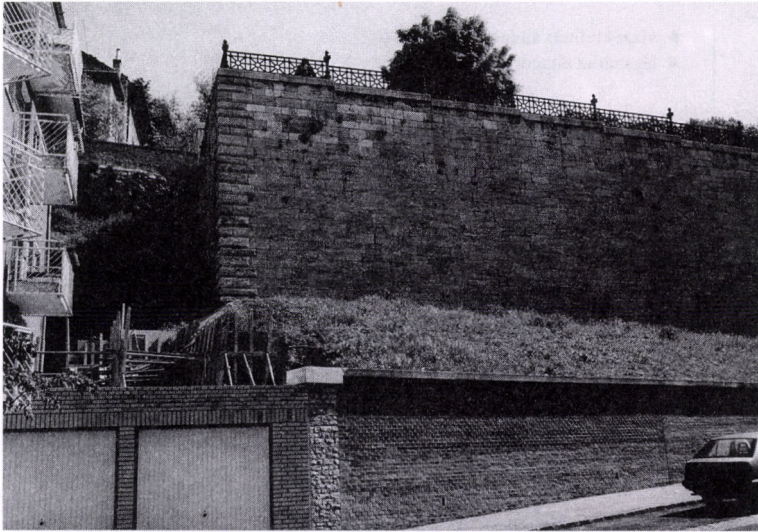
2. kép. A Tábor utcai támfal
