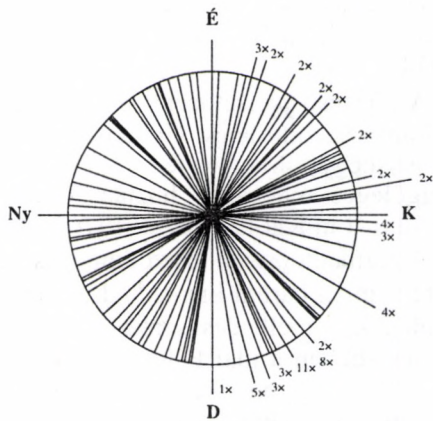
2.9. ábra. Az édesvízi mészkő köztréseinek gyakoriság diagramja, Polgárváros D-i része
