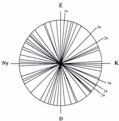
2.10. ábra. Az édesvízi mészkő litoklázisainak gyakoriság diagramja, Polgárváros
