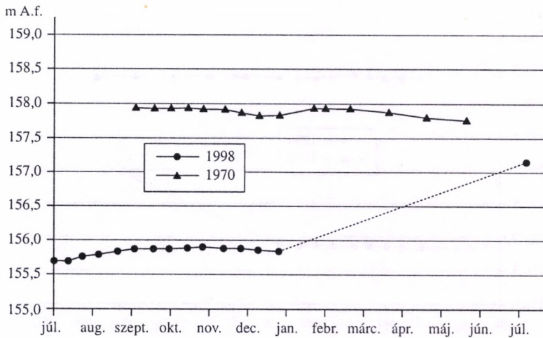
3.16. ábra. A Német kút vízállás-idősorai
