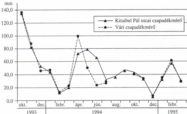
4.1. ábra. Havi csapadék adatok összehasonlítása
