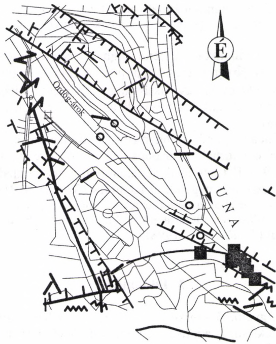
2.6. ábra. A budai Várhegy környezetének tektonikája (WEIN 1974 nyomán)
