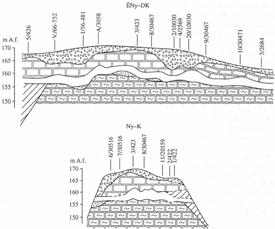
2.5. ábra. Vázlatos földtani szelvény (A metszetek nyomvonalát 2-es számú mellékleten látható.)
