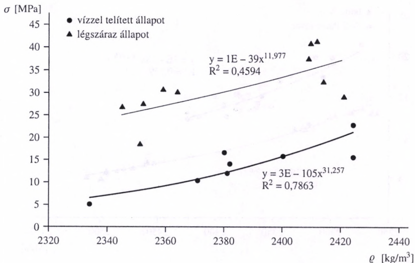
3.2. ábra. A budai márga testsűrűség-nyomószilárdság diagramja
