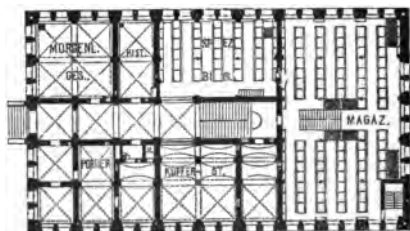
Földszint.
