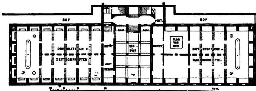
(Földszint.)
