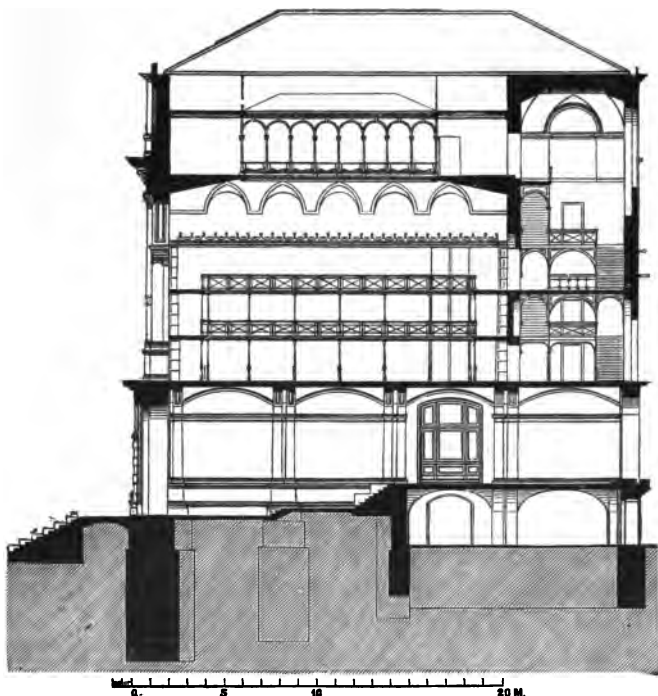
32. kép. Királyi és országos könyvtár Stuttgartban.
