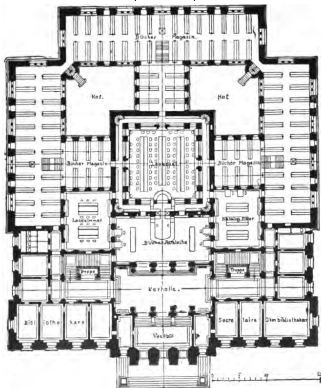
(Földszint.)
