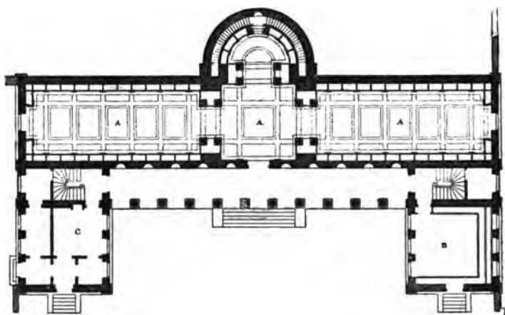
14. kép. Nyilvános könyvtár Amiensban. (Alaprajz. — \frac{1}{600} -hoz.) A. Könyvterem. B. Olvasóterem. C. Könyvtárnok lakása.
