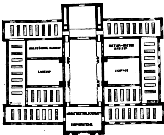
(Emelet.)
