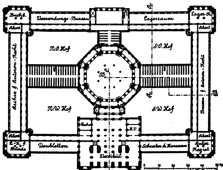
(Földszint.)
