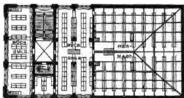
II. emelet.
