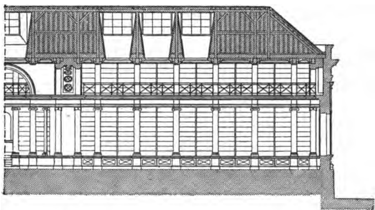
16. kép. Nyilvános könyvtár Amiensban. (Hosszmetszet. — \frac{1}{250} -hez.)
