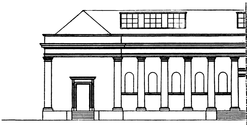
15. kép. Nyilvános könyvtár Amiensban. (Külső kép. — \frac{1}{250} -hez.)
