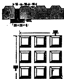
86. kép. Üvegpadló részlet a Reichstagsbibliothekből Berlinben.
