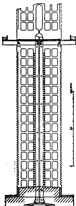
Könyvpolcz, könyvtartó s a könyvállvány oldalnézete a fog- és csapberendezéssel.
