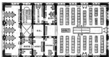
I. emelet.
