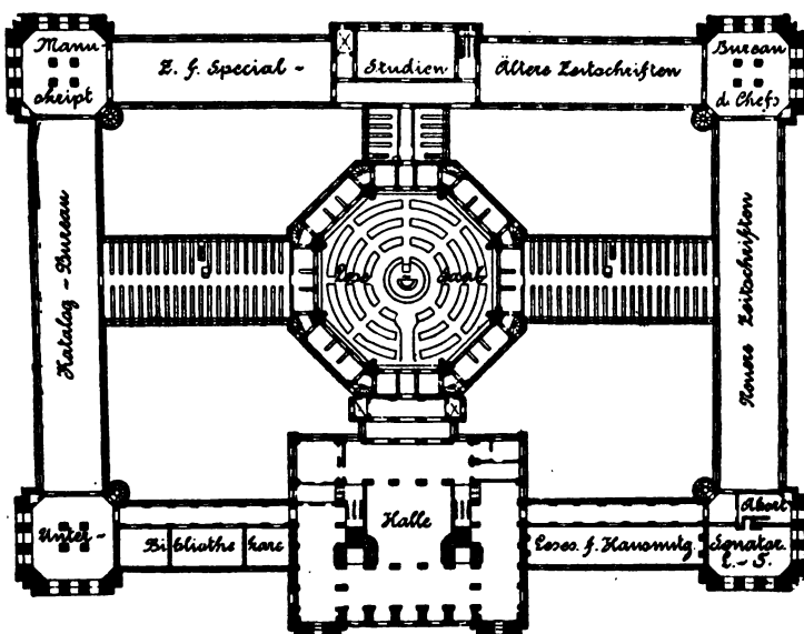
(I. emelet)
