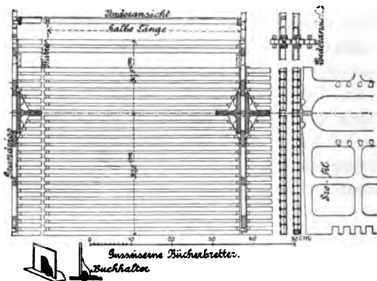
Könyvpolcz, könyvtartó s a könyvállvány oldalnézete a fog- és csapberendezéssel.
