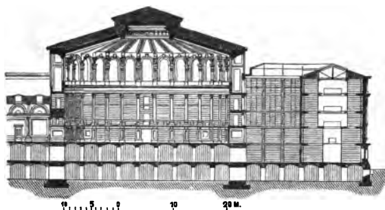
(Keresztmetszet.)
