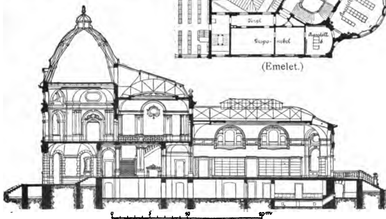
Metszet az előépítményen át.
