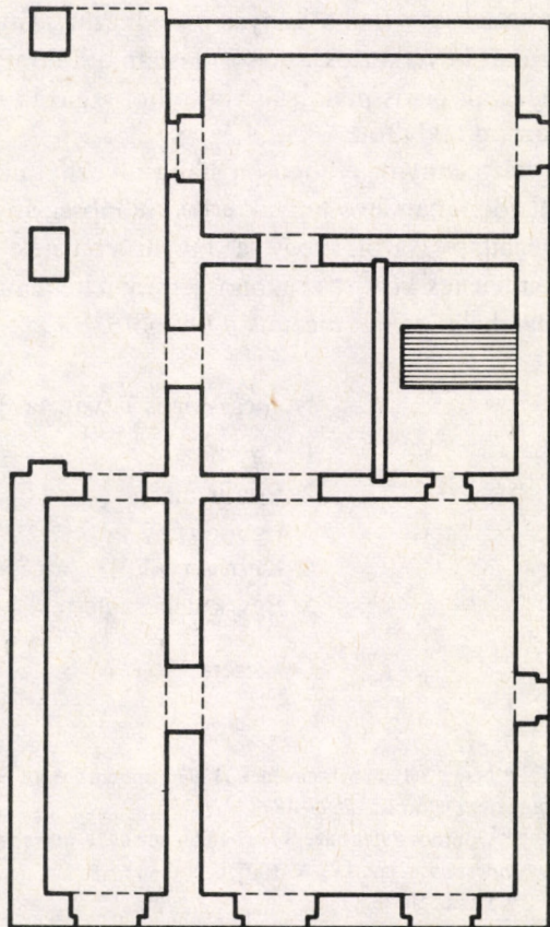
1. ábra nemes Harangi György debreceni lakos Varga utcai házának tervrajza, 1820.
