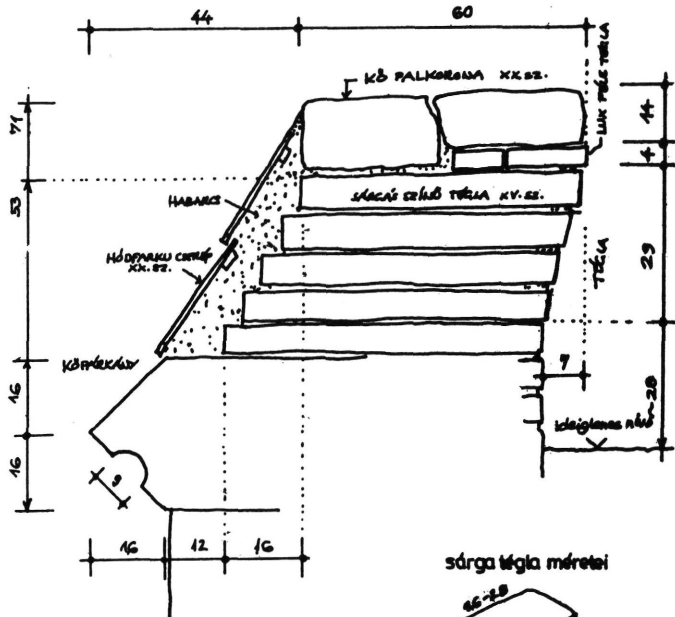
① METSZET
